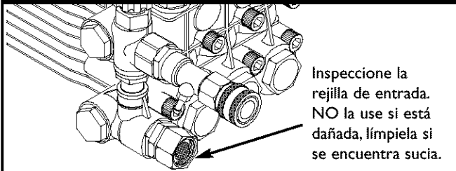
Figura 18 - Conecte la Manguera para el Jardín, a la Entrada de Agua
