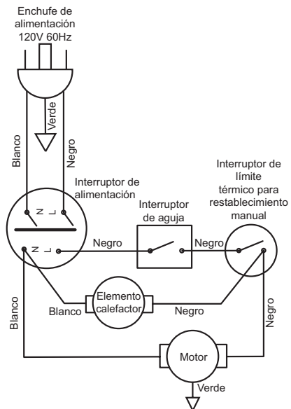
Figura 4. Restablecimiento del interruptor de límite térmico
