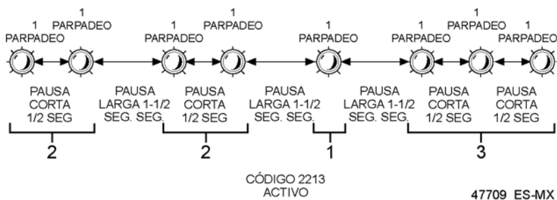
Figure 17 Ejemplo Código de Destello de RSL (Apagar el Motor)
