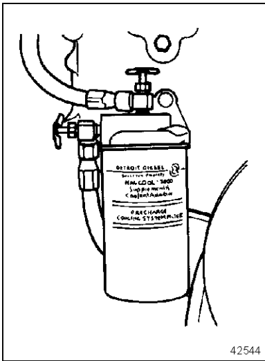
Figure 28 Elemento inhibidor del líquido refrigerante
