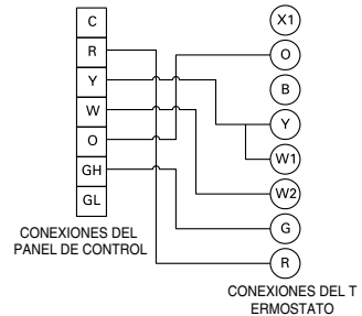
Esquema del cableado de la unidad de refrigeración recta.
