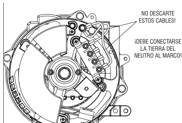
Figura 7 - Conexión A Tierra Del Neutro Al Marcos
