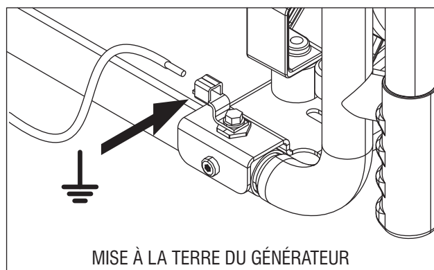
Schéma 6 - Mise à la terre du générateur
