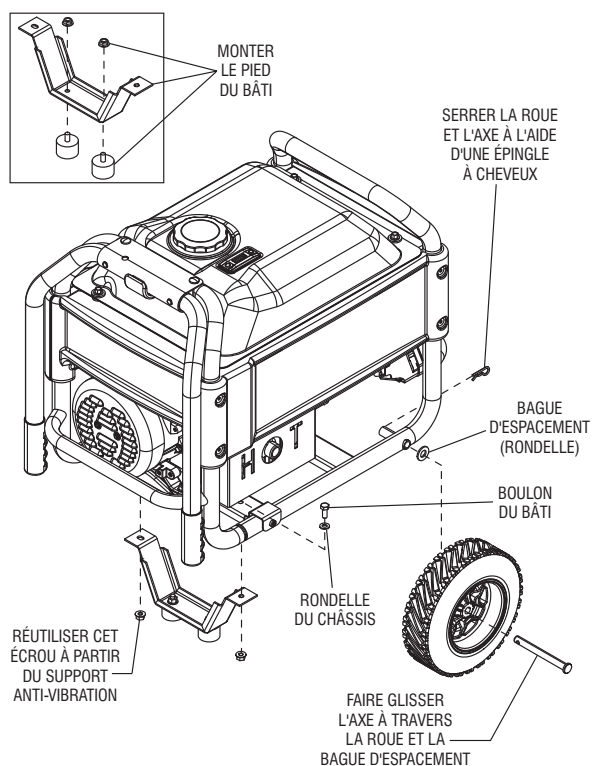
Schéma 2 – Montage de la roue
