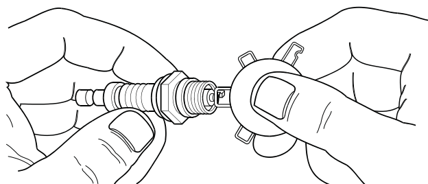
Schéma 12 - Écartement de la bougie d'allumage
