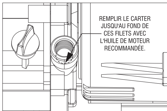
Schéma 8 - Le niveau d'huile
