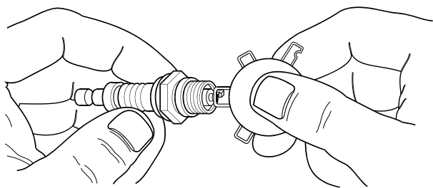
Figura 12 - Espaciamento de la bujía.
