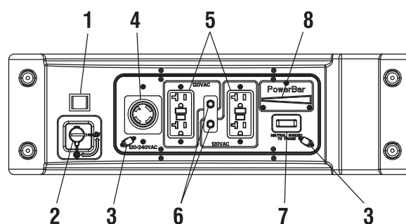
Figura 3 - Controles del generador
