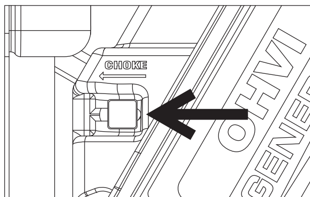
Figura 11 - Posición de Choke
