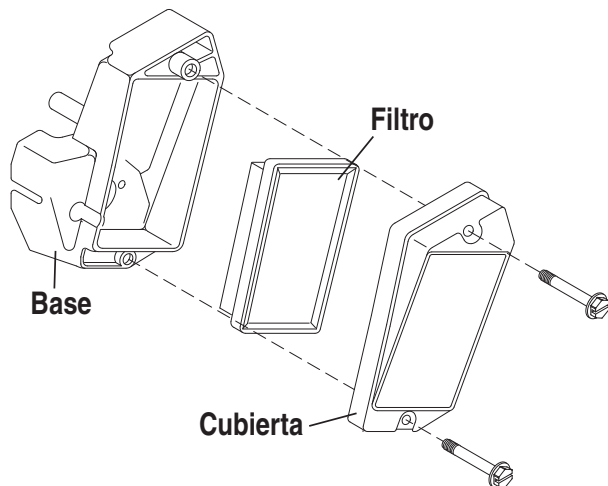
Figura 13 - Limpiador de aire
