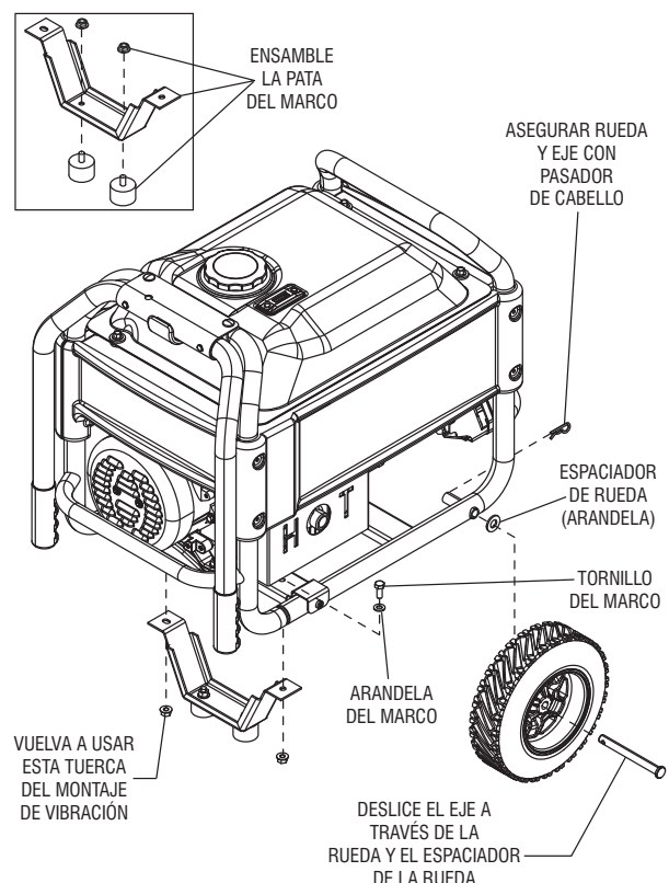
Figura 2 – Rueda y La Plata Del Marco
