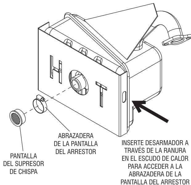
Figura 14 - Supresor de chispa
