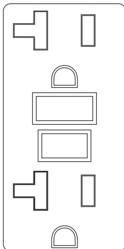
Figura 4 - Receptáculo dúplex GFCI de 120 Volt AC, 20 Amp
