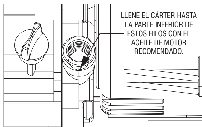
Figura 8 - Del nivel de aceite
