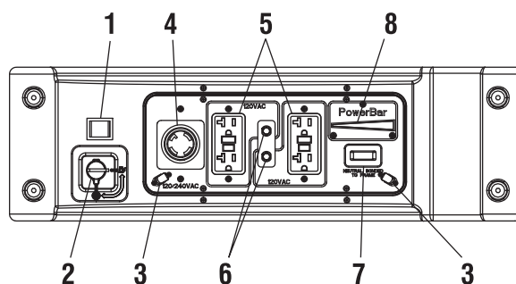
Schéma 3 - Commandes du générateur
