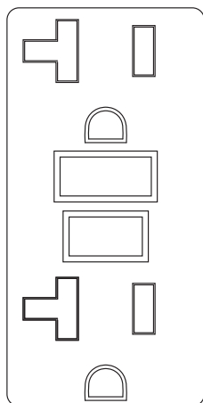
Schéma 4 - Prise double DDFT, 120 V c.a., 20 A
