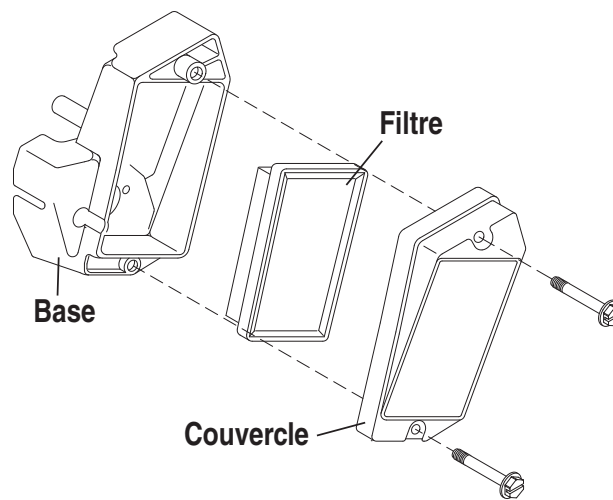
Schéma 13 - Filtre à air
