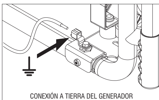
Figura 6 - Conexión a tierra del generador
