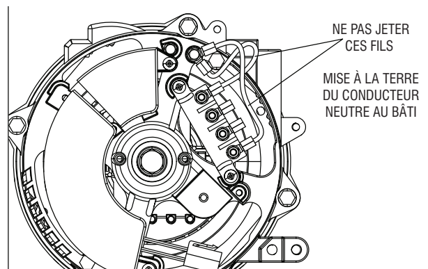
Schéma 7 - Mise à la terre du conducteur neutre au bâti
