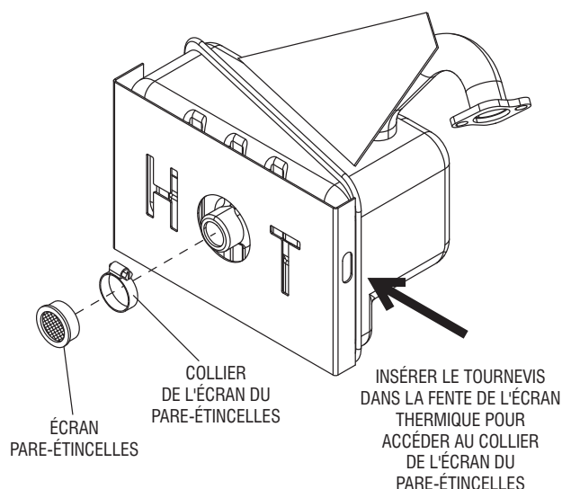
Schéma 14 - Pare-étincelles
