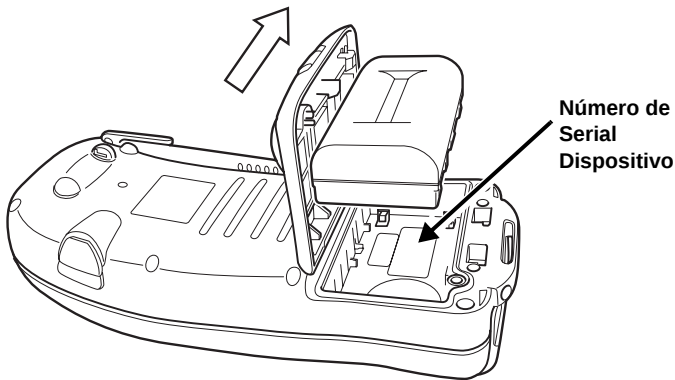
Figure 2-4. Instalación de la Batería Primaria
