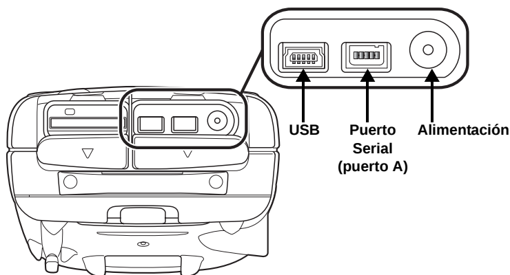
Figura 1-5. Puertos GMS-2
