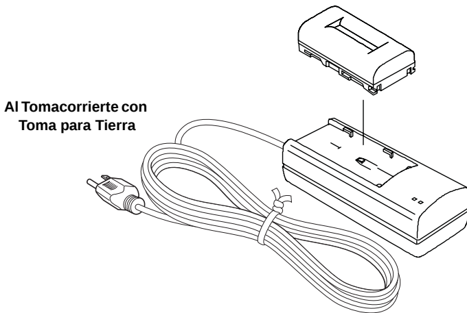
Figure 2-3. Carga de la Batería en el Cargador
