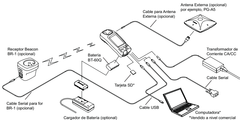
Figure 3-1. Conexiones del Sistema GMS-2
