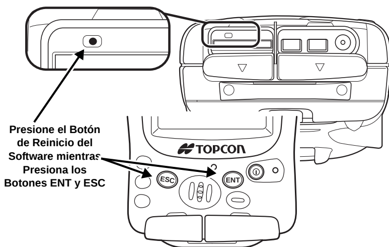
Figura 4-2. Reinicio del Hardware
