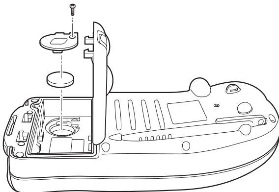
Figure 2-5. Cambio de la Batería Tipo Botón
