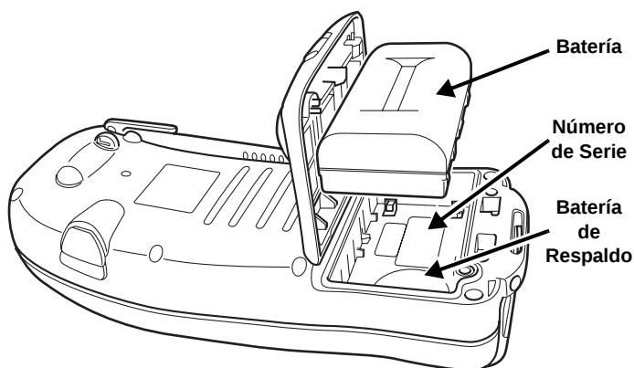
Figura 1-2. Batería del GMS-2
