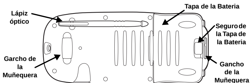
Figura 1-4. Parte Posterior del GMS-2
