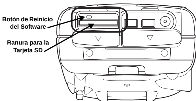
Figura 1-6. Ranura de la Tarjeta SD
