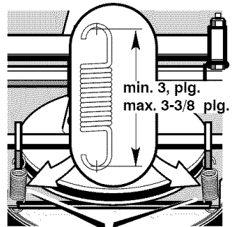
Resorte de propulsión Figura 93
