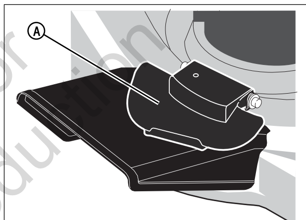
Figura 10: Liberación de la cubierta del triturador
