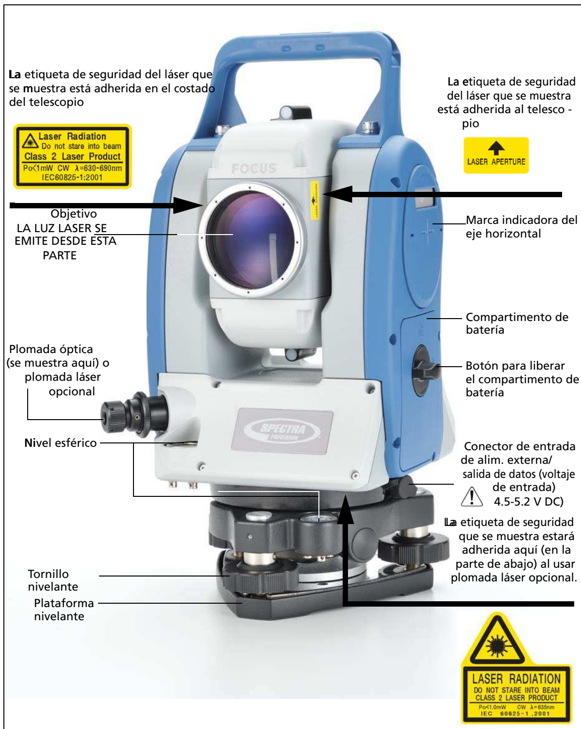
Figura 3.2 Vista frontal de la estación total Focus 6 de 5" (Cara izquierda)
