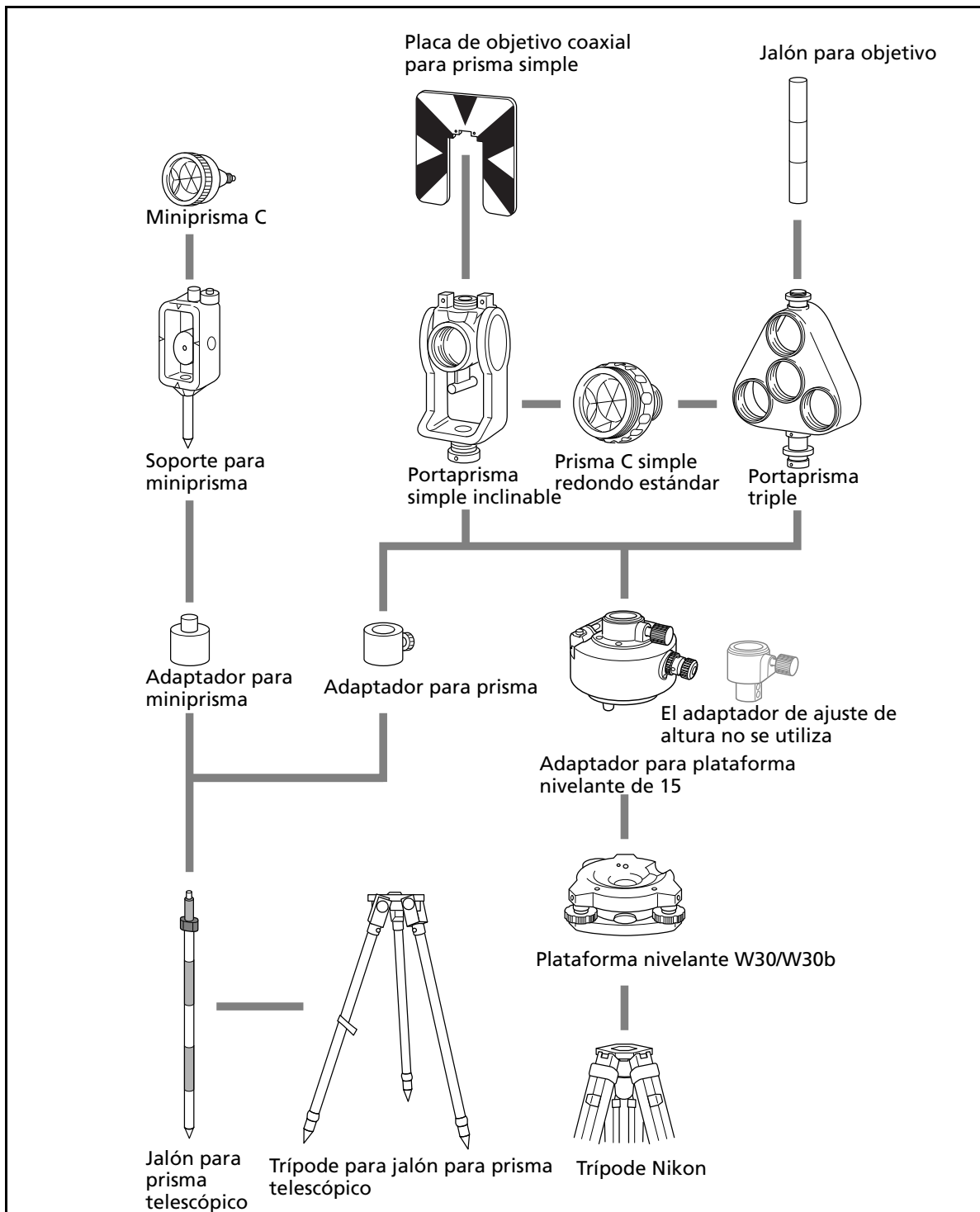
Figure 8.2 Lado con el prisma reflector
