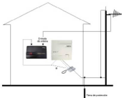
ITC 4000 con mástil o torre
