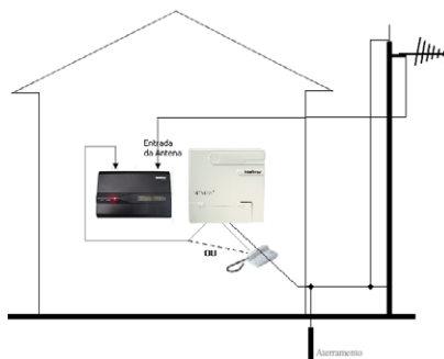
ITC 4000 com mastro ou torre
