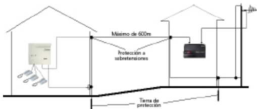
Instalación de la ITC 4000 en abrigo externo
