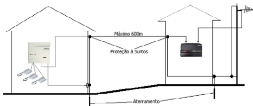
Instalação da ITC 4000 em abrigo externo
