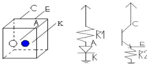
Figura 8. Configuración del Sensor CNY70
