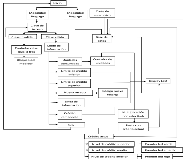
Figura 9. Diagrama de flujo del programa
