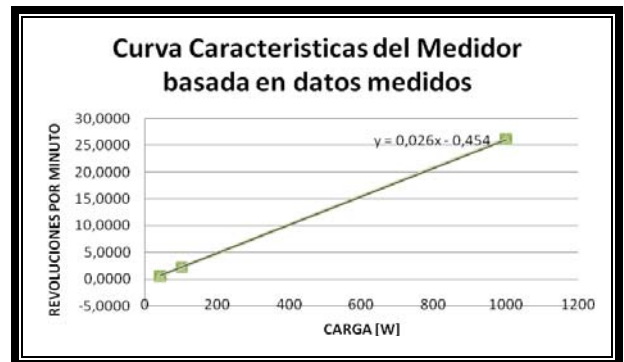
Figura 5. Curva característica del medidor.
