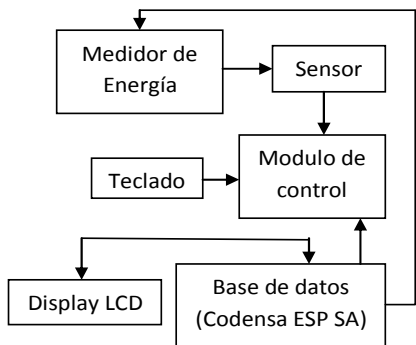
Figura 7. Diagrama de Bloques del sistema
