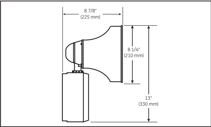
Figura 1. Dimensiones
