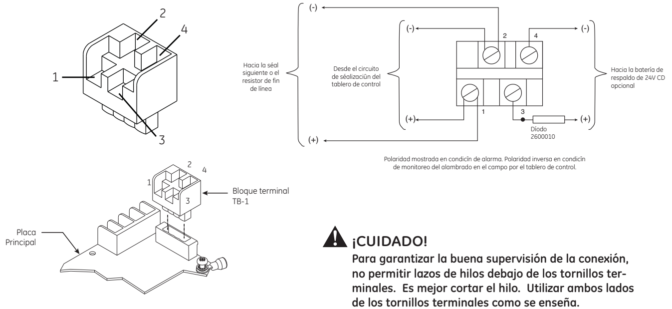
Figura 3. Alambrado al bloque terminal BT1
