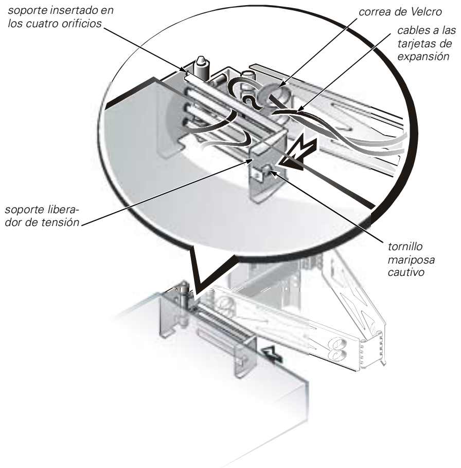
Figura 4-12. Cómo acoplar el soporte de liberación de tensión
