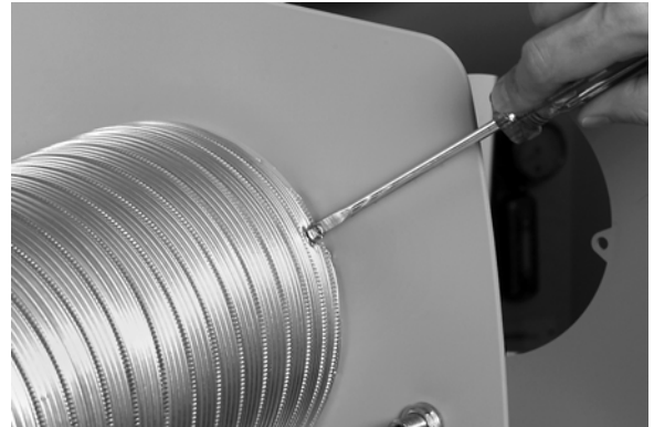
Fig. 14. Raccordement de la gaine de dérivation à l'humidificateur.
