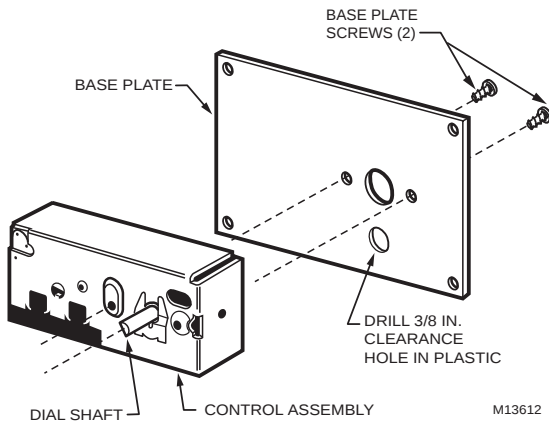
Fig. 45. Mounting Humidistat.
