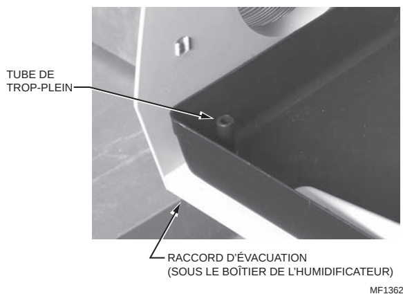
Fig. 28. Installation du bac d'eau.
