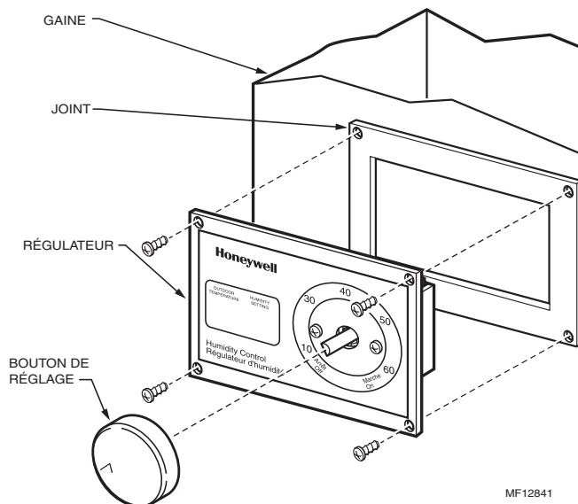
Fig. 42. Fixation de l'humidistat sur la gaine.
