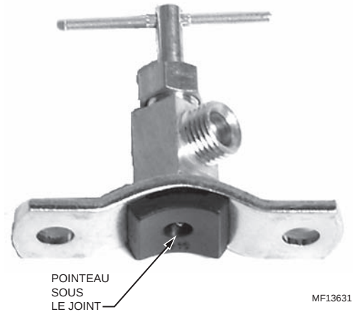
Fig. 31. Ajustement du robinet-vanne à étrier dans une installation sur un tuyau en cuivre.
