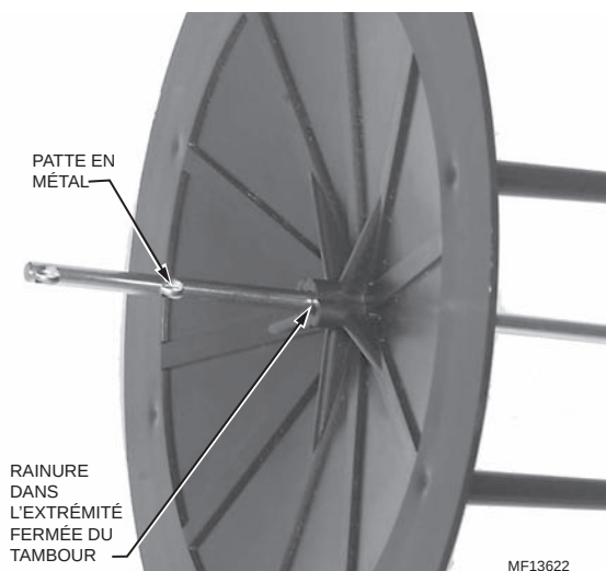
Fig. 16. Assemblage de l'extrémité fermée du tambour.
