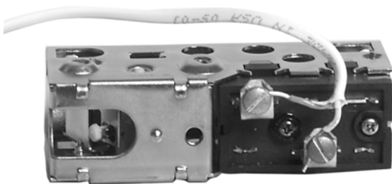
Fig. 41. Wiring Humidistat.
