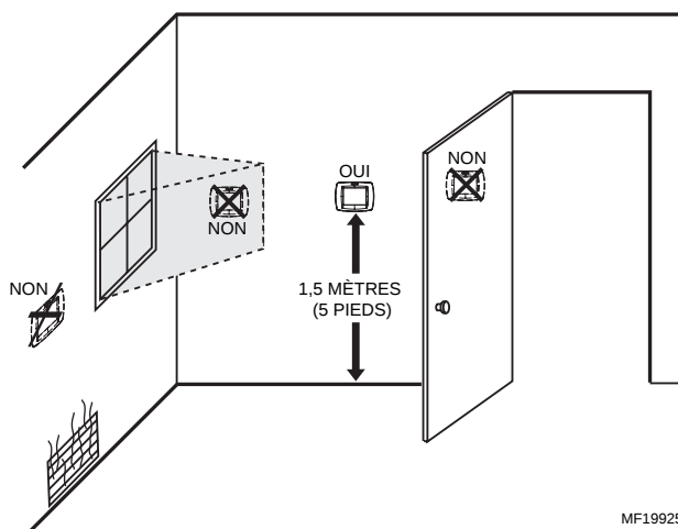
Fig. 43. Choix de l'emplacement de l'humidistat.
