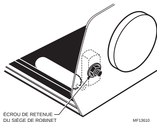
Fig. 23. Écrou de retenue du robinet à flotteur.
