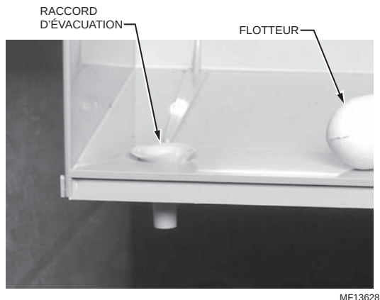
Fig. 27. Installation du raccord d'évacuation.
