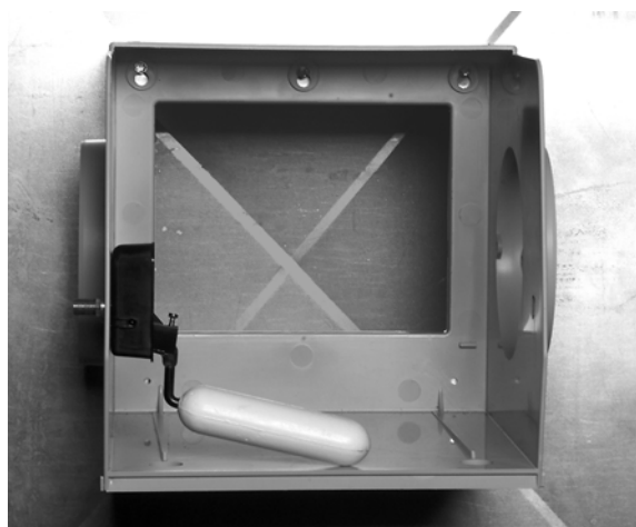
Fig. 7. Montage de l'humidificateur.
