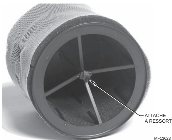
Fig. 19. Installation de l'extrémité ouverte du tambour.
