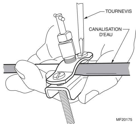
Fig. 32. Installation du robinet-vanne à étrier.
