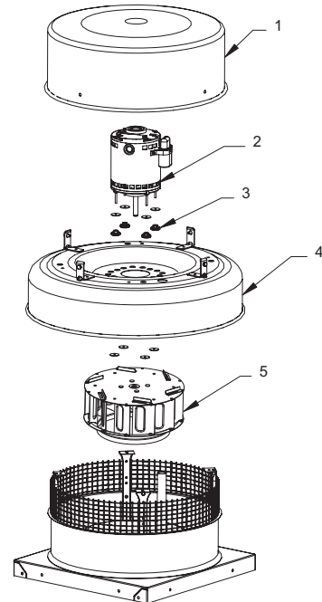
Figure 5 — Pièces de rechange pour tourelles d'extraction à jet descendant centrifuges à entraînement direct
