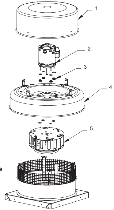
Figura 5 — Ilustración de Repuestos para Extractores Centrífugos de Transmisión Directa de Tiro Hacia Abajo
