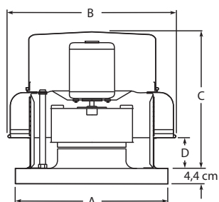
Figura 1 — Dimensiones
