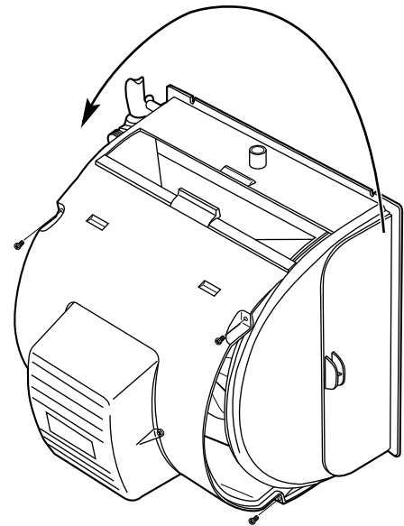
Fig. 8—Reversing Door Access on HUMBBSFP1016-A--
