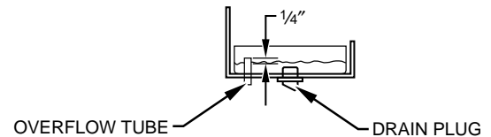
Fig. 16—Water Level in HUMBWTR2019-A--
