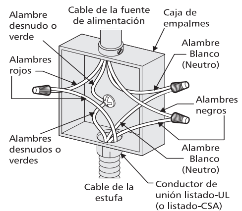
Figura 6 - Sistema eléctrico de 4 alambres (ejemplo caja de empalmes)
