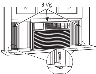
2 ferrures de verrouillage de cadre
