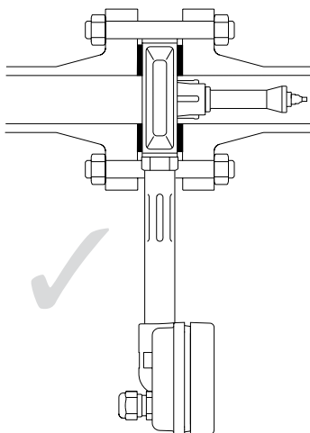
Fig. 16 Juntas montadas correctamente
