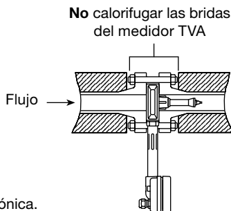
Fig. 6 Calorifugado de la línea
