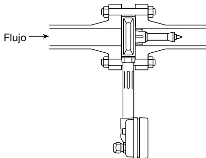
Fig. 9 Flujo Horizontal hasta 32 bar r
