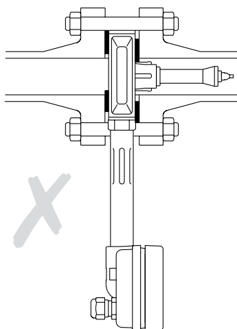
Fig. 17 Juntas montadas incorrectamente
