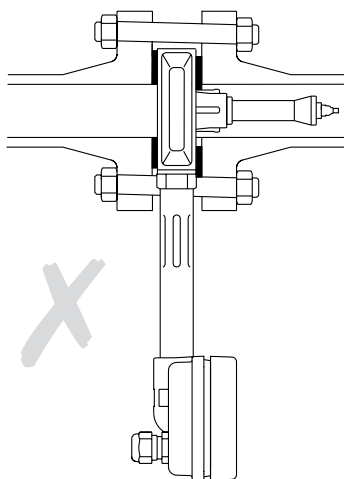
Fig. 18 Juntas y tubería descentradas, montaje incorrecto
