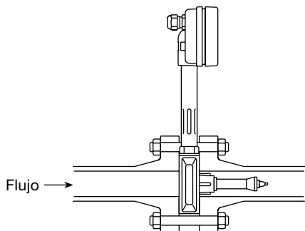
Fig. 8 Flujo Horizontal limitado a 7 bar r
