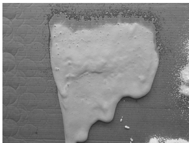
A-rich Foam
