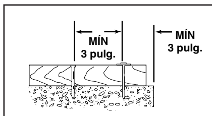
ESPACIO: FRANJA DE MADERA DELGADA A CONCRETO
