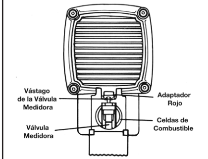
Vista cenital de la herramienta TrakFast
