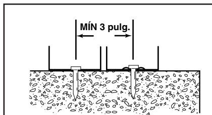
ESPACIO: METAL DE CALIBRE DELGADO A CONCRETO
