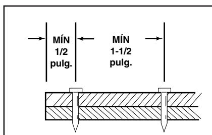
ESPACIO ACERO A ACERO
