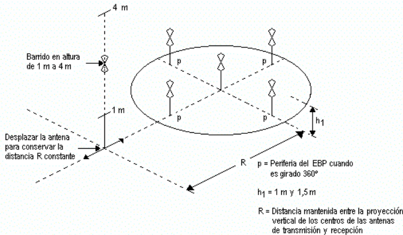
Figura A.3.- Polarización horizontal y vertical
