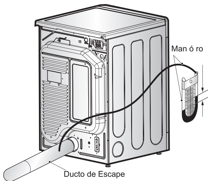
Medición de la Presión Estática.
