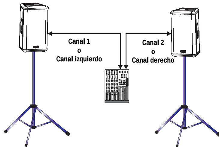
Diagrama físico del ejemplo de aplicación N°1.
