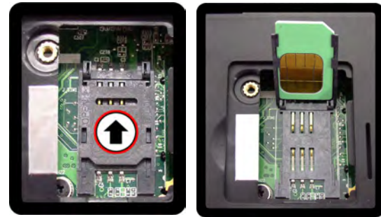
Figura 10 - Desbloquear SIMLOCK
