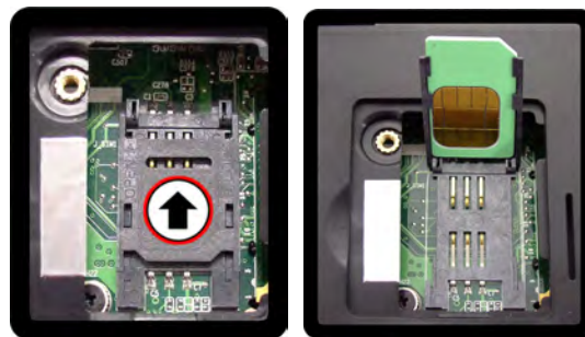
Abb. 10 - Lösen des SIMLOCK-Riegels
