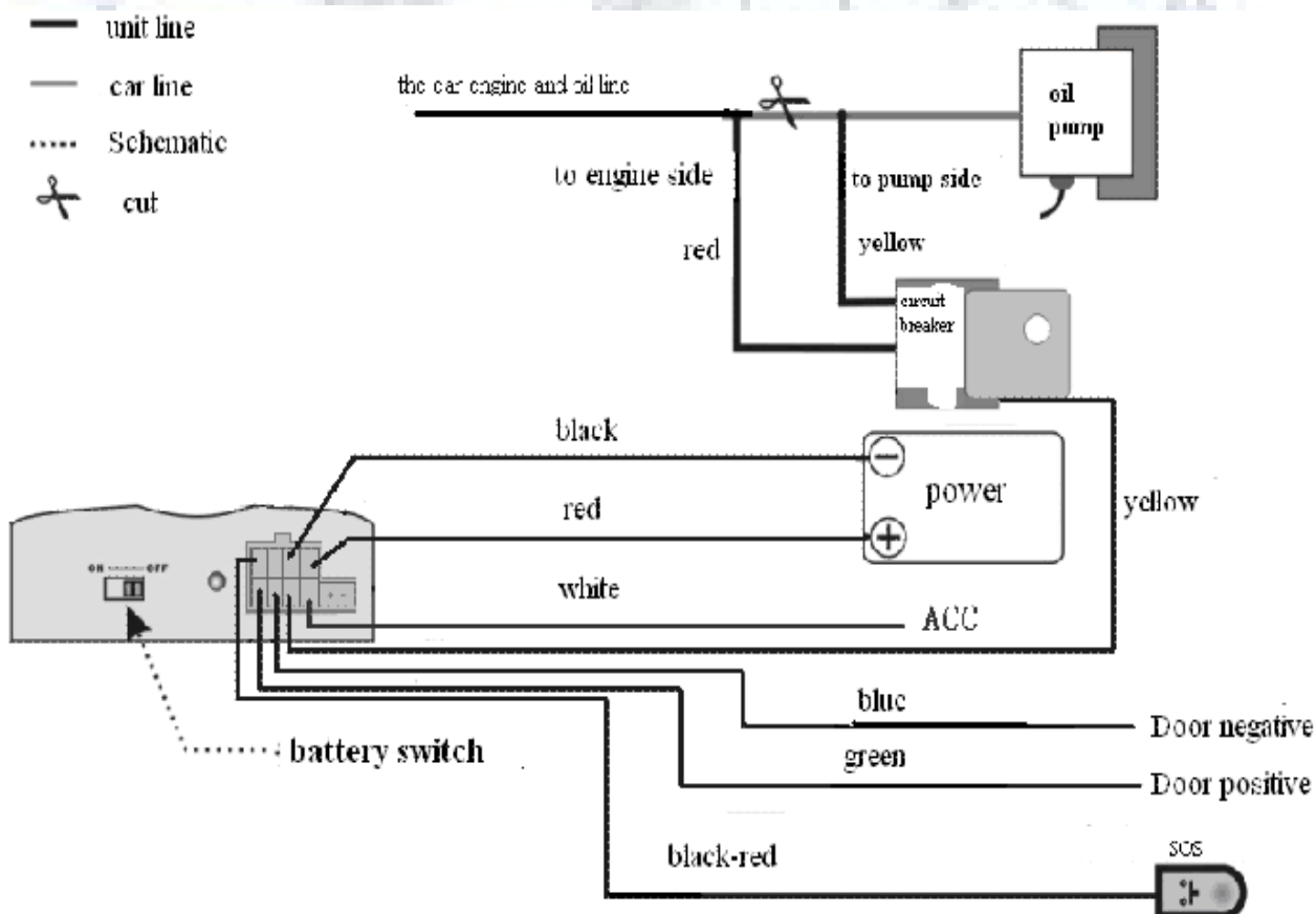
Figura 6 - Schema collegamenti
