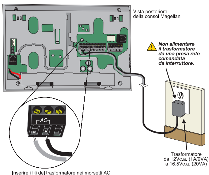
Figura 1. Connessione del trasformatore
