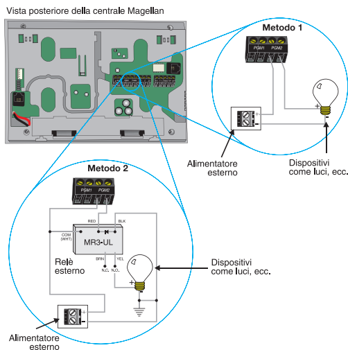
Figura 6. Connessioni PGM
