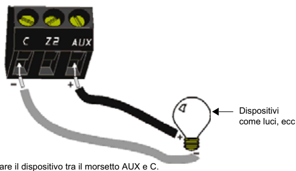
Figura 3: Collegamenti Uscita Ausiliaria
