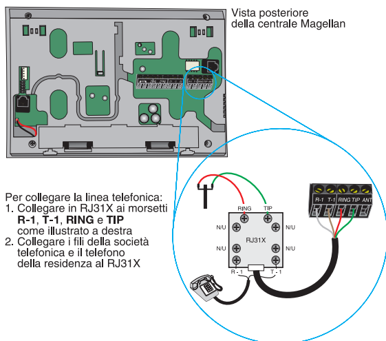
Figura 4. Connessione diretta della linea telefonica
