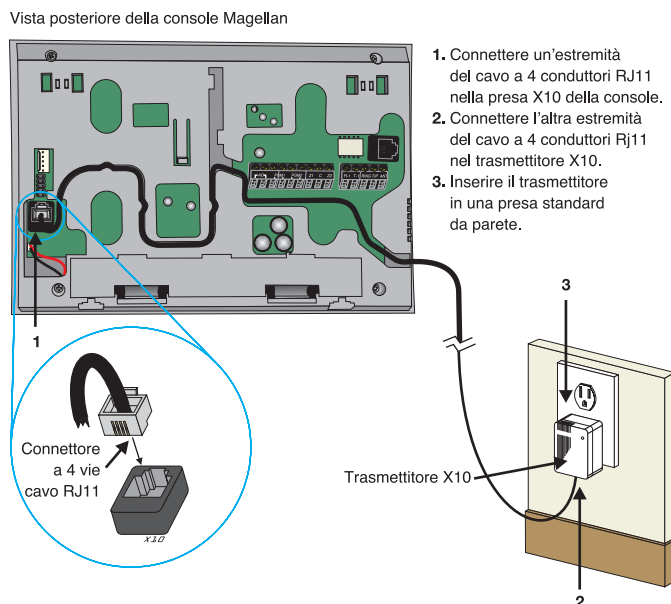
Figura 9. Connessione trasmettitore X10
