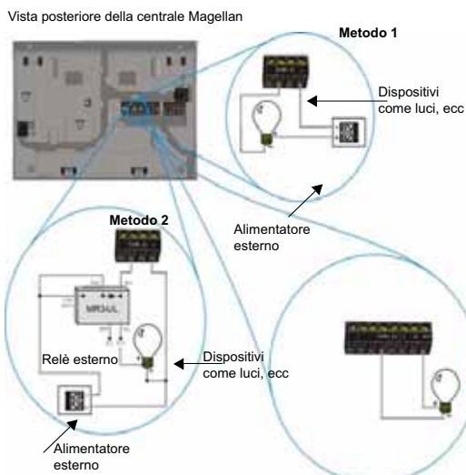
i Figura 7. Collegamenti PGM2
