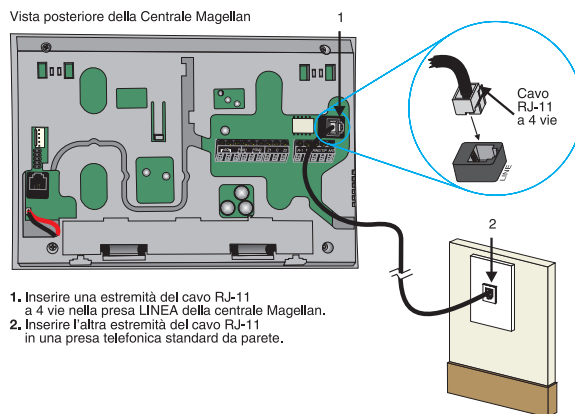
Figura 5. Connessione presa di linea
