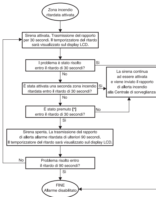
Figura 18. Zona incendio ritardata
