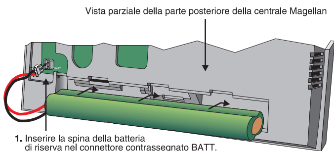
Figura 2. Connessione della batteria di riserva
