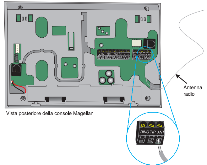
Figura 15. Connessione dell'antenna radio
