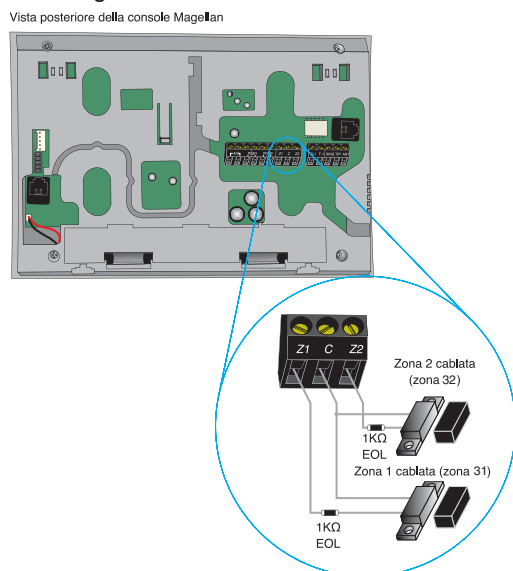
Figura 8. Connessioni zone cablate
