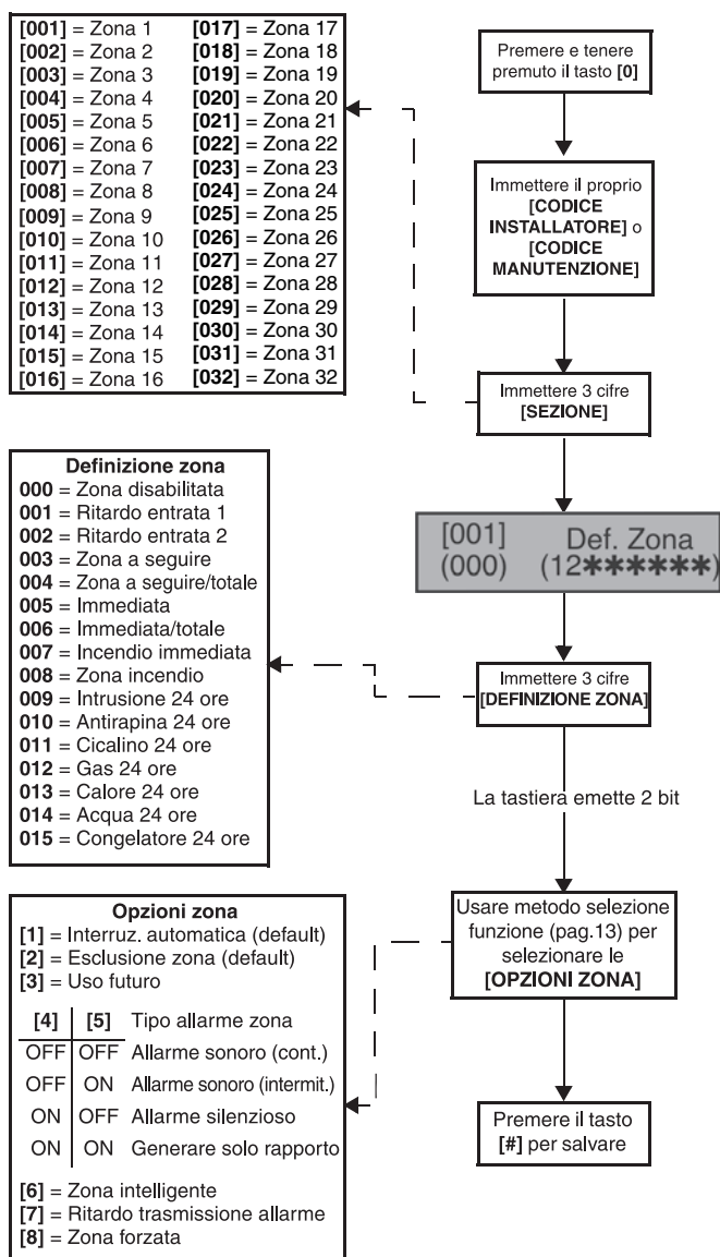
Figura 14. Generalità sulla programmazione zone di Magellan
