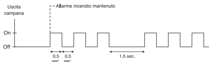
Figura 17. Uscita campana/sirena durante un allarme incendio
