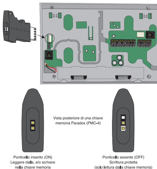
Figura 10. Connessione di una chiave memoria Paradox (PMC-4)
