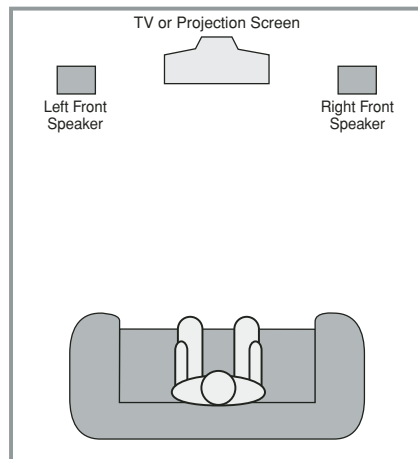
B) La distanza tra i diffusori sinistro e destro deve essere uguale a quella fra la posizione d'ascolto seduta e lo schermo.
