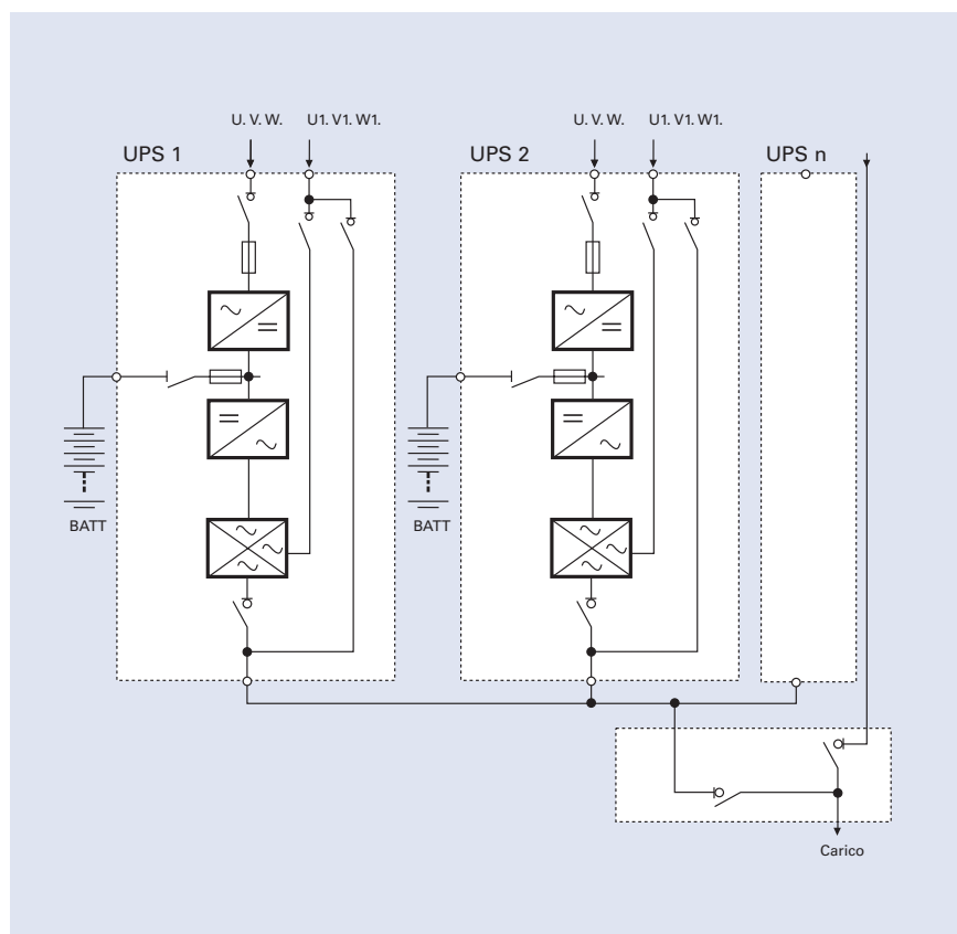
Figura 6. Configurazione di Parallelo Modulare
