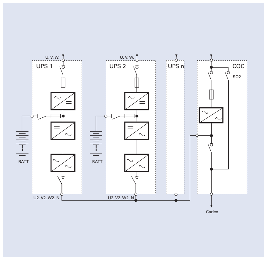
Figura 7. Configurazioni in parallelo con modulo centrale di distribuzione (COC)
