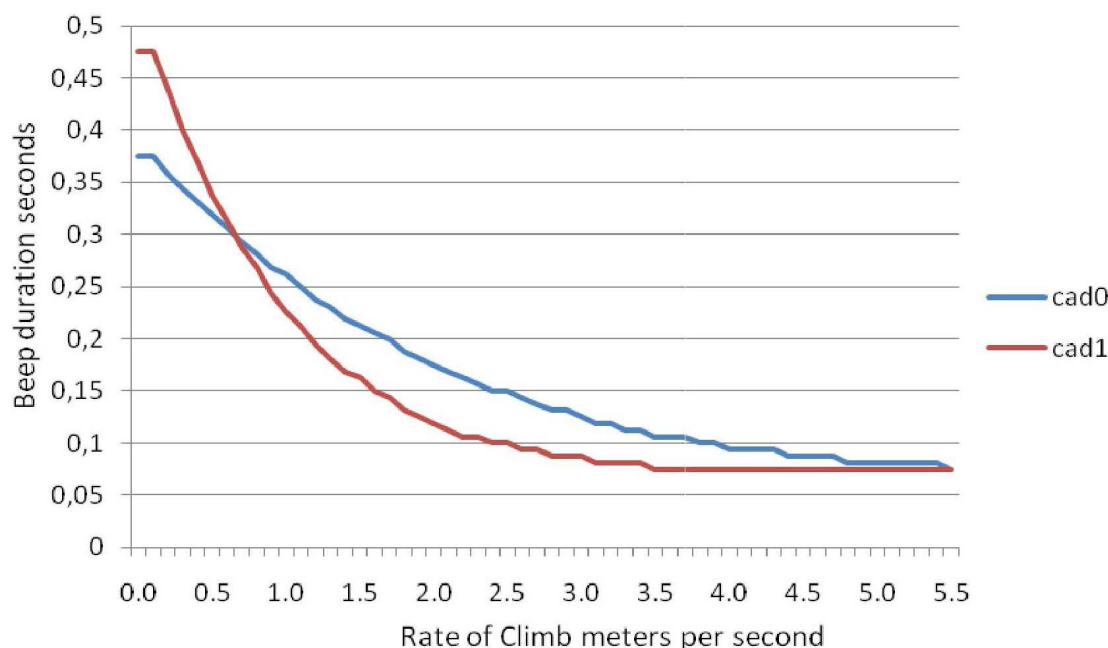
Figura 31 – Curve di incremento della cadenza
