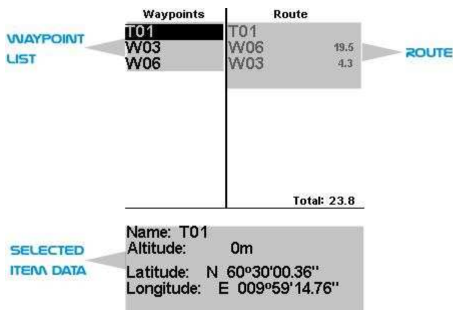
Figura 17 – Pagina impostazioni waypoint e task
