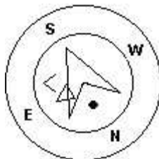
Figura 9 - Posizione del nocciolo (o core) della termica
