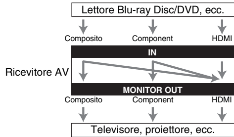
Diagramma di flusso del segnale video
