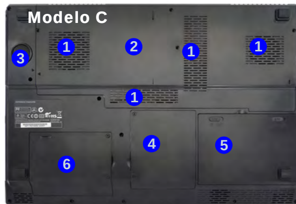
Figura 9 Vistas inferior
