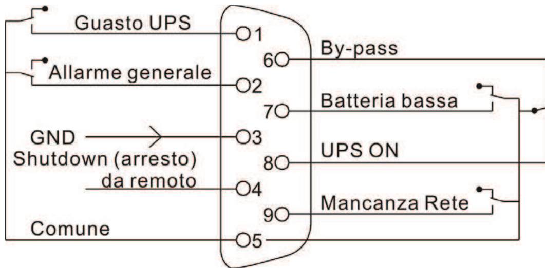
Interfaccia DB-9 del protocollo di comunicazione AS400
