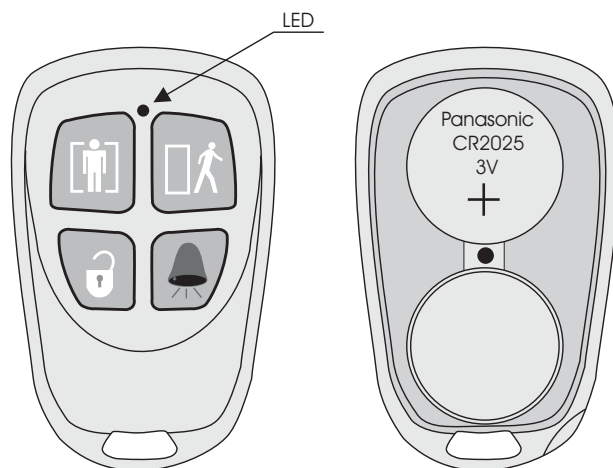
Figura 5 Radiochiave
