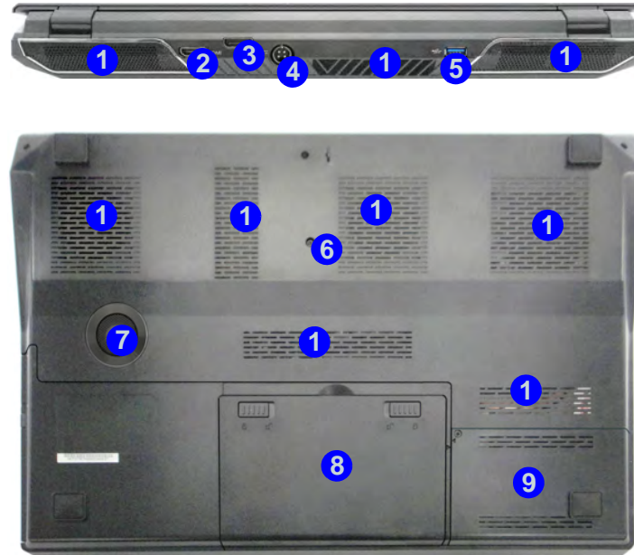
Abb. 8 - Ansicht von hinten und unten
