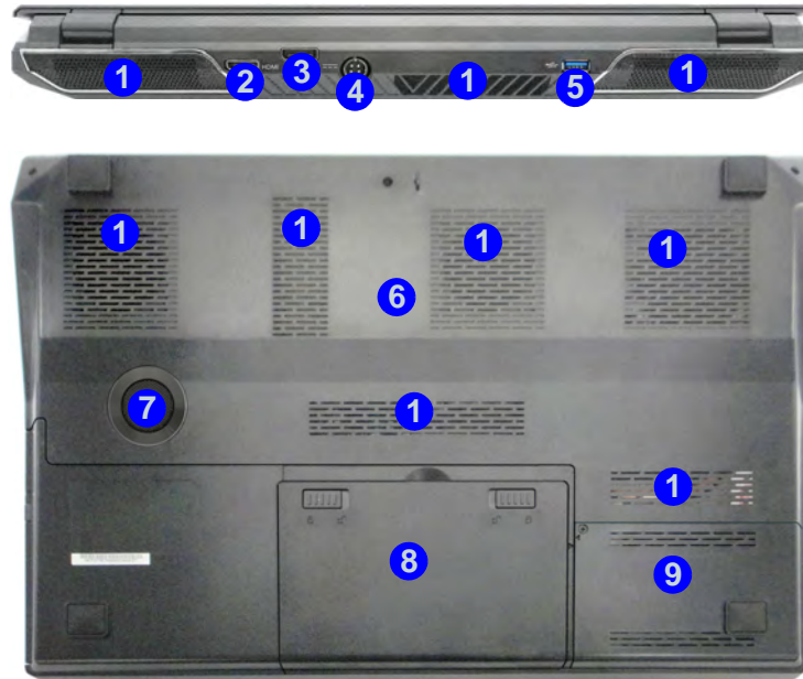
Figura 8 - Vistas posterior y inferior
