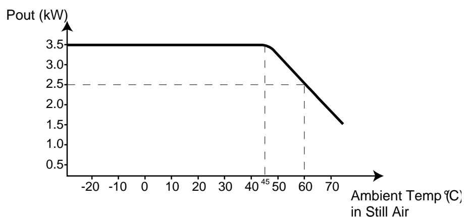
Figura A-1 Potenza di uscita rispetto alla temperatura ambiente
