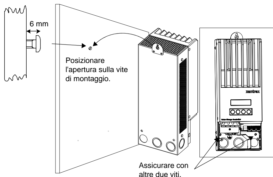
Figura 2-5 Montare il Regolatore di carica solare XW
