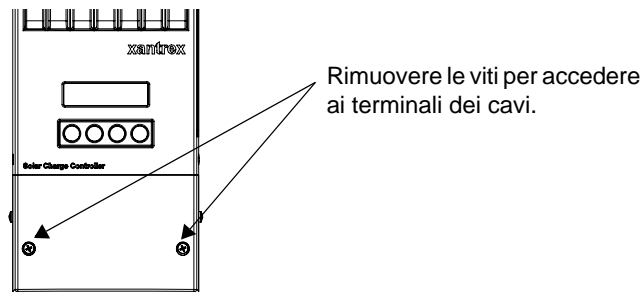
Figura 2-2 Rimozione del pannello dello scomparto dei cavi
