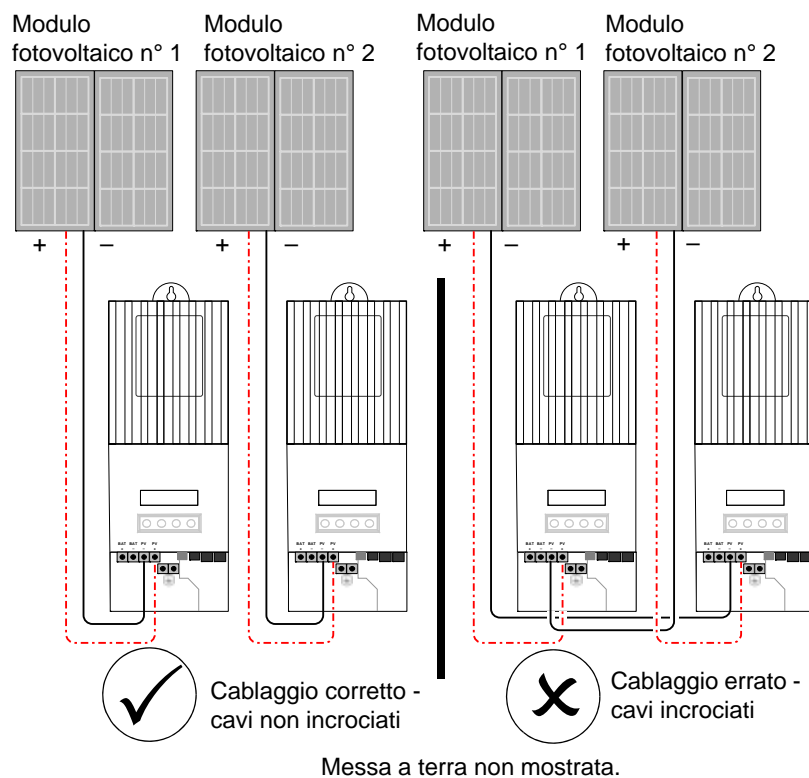
Figura 2-10 Cablaggio XW SCCmultiplo CC
