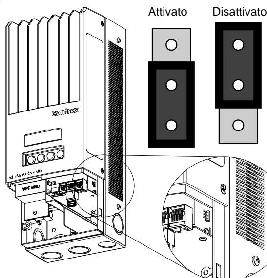
Figura 2-7 Posizione del connettore di messa a terra negativo
