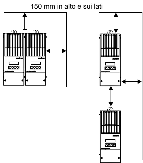
Figura 2-1 Requisiti minimi di spazio libero
