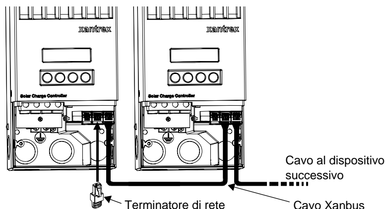
Figura 2-12 Struttura della rete
