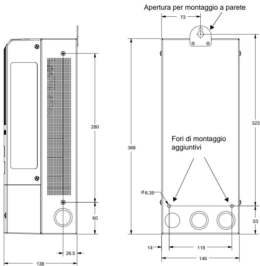
Figura 2-3 Dimensioni e posizione dei knockout
