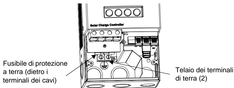
Figura 2-6 XW SCC Connettore a terra di sicurezza
