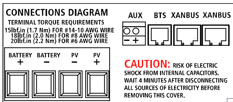
Figura 2-8 Terminali di connessione CC
