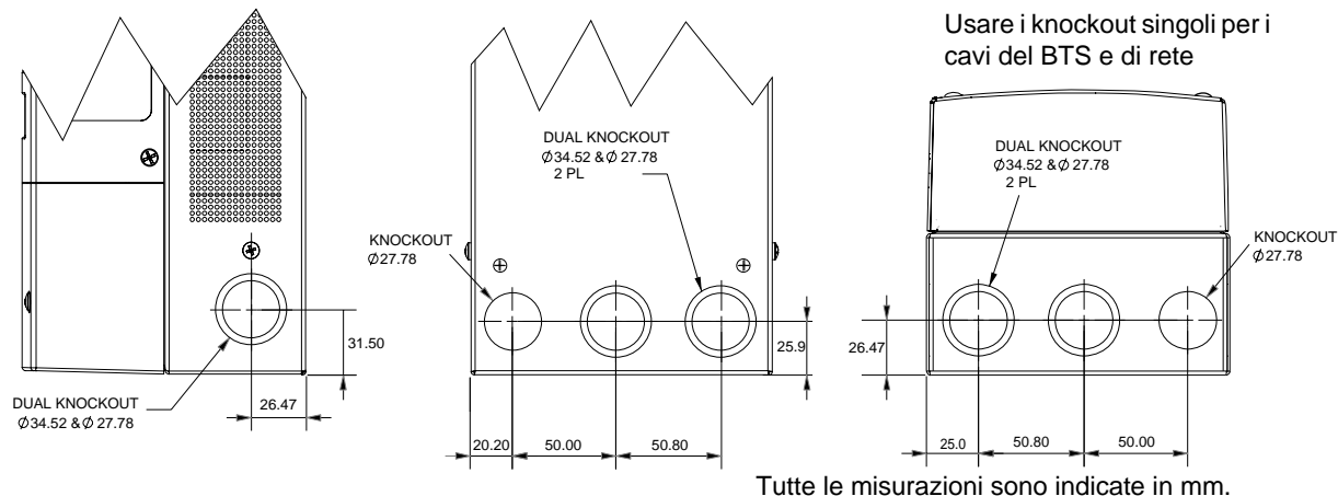
Figura 2-4 Dimensioni dei knockout
