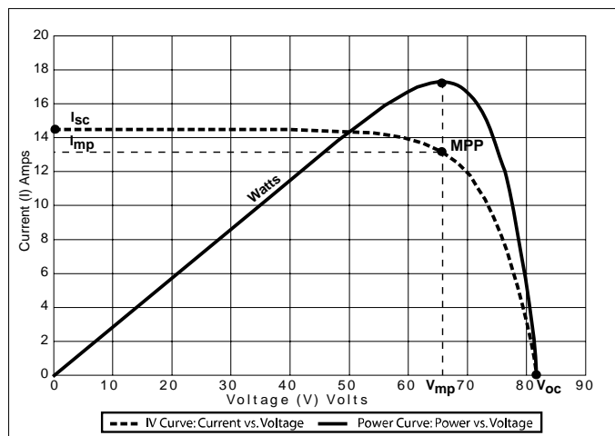
Figura 1-1 Curva del punto di massima potenza
