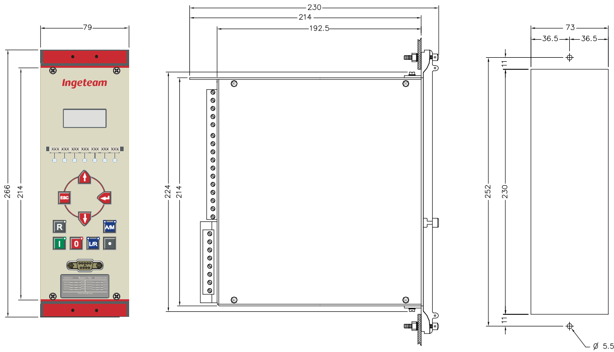
-Dimensioni PL70FV
