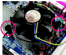
Fig. 3 Mettere il dissipatore di calore sopra la CPU e assicurarsi che i push pins siano in direzione dei fori dei pin hole sulla scheda madre. Premere verso il basso i push pins in diagonale.
