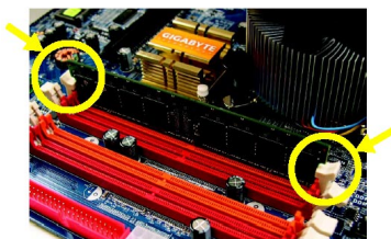
Fig. 2 Chiudere le clip di plastica su entrambi i lati del socket DIMM per bloccare il modulo DIMM. Seguire i passi dell'installazione al contrario nel caso si volesse rimuovere i banchi di memoria DIMM.
