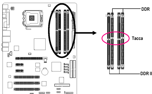
Fig. 1 Il socket DIMM ha una tacca di inserimento, così il modulo di memoria DIMM può essere inserito solo in una direzione. Inserire il modulo di memoria DIMM verticalmente nella relativa presa. Quindi premere verso il basso.
