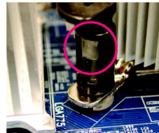
Fig. 4 Assicurarsi che i push pin maschio e femmina siano saldamente uniti. (per le istruzioni dettagliate sull'installazione, fare riferimento alla sezione sull'installazione del dissipatore di calore del manuale dell'utente)
