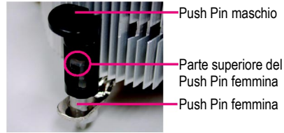
Fig. 2 (Girando il push pin verso la direzione della freccia per rimuovere il dissipatore di calore, in senso contrario per installarlo.) Fare attenzione che la direzione della freccia sul push pin maschio non siano rivolte verso l'interno prima dell'installazione. (Questa istruzione è valida solo per ventilatore incorporato Intel)
