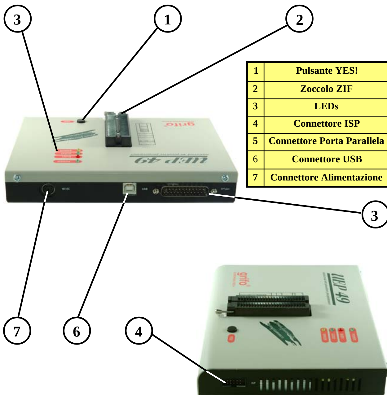
FIGURA 9: POSIZIONE DI CONNETTORI, LEDs, ECC.
