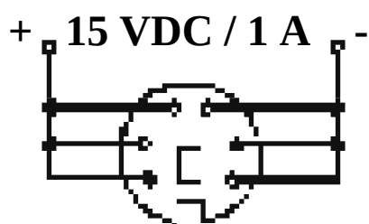
FIGURA 10: CONNETTORE DI ALIMENTAZIONE
