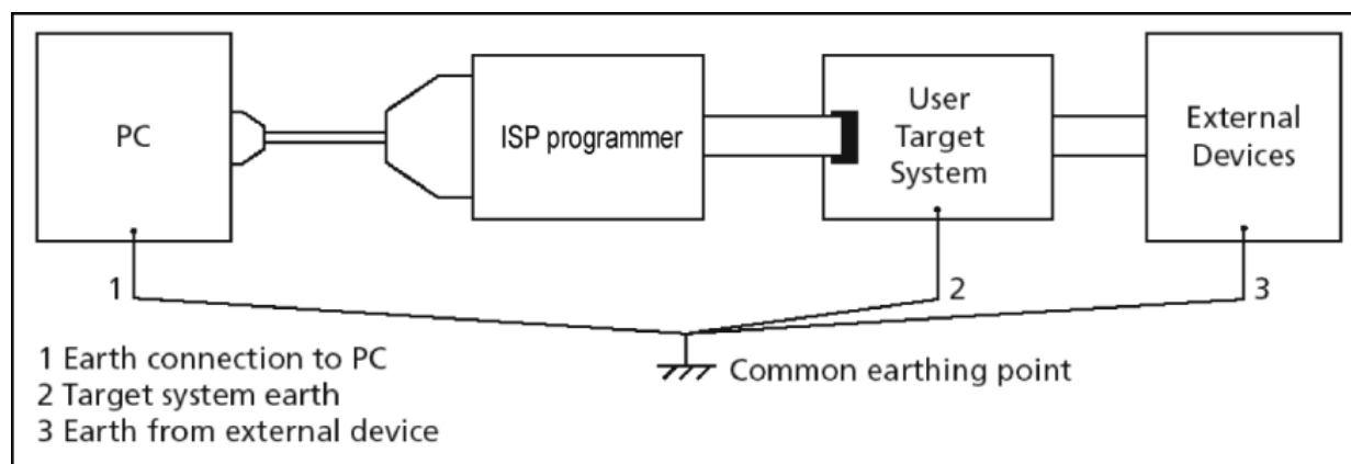
FIGURA 3: ESEMPIO DI CONNESSIONE ISP
