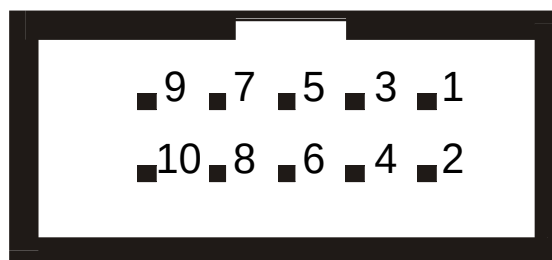
FIGURA 5: CONNETTORE ISP DI UEP 49
