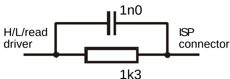
FIGURA 4: DRIVER ISP DI UEP 49
