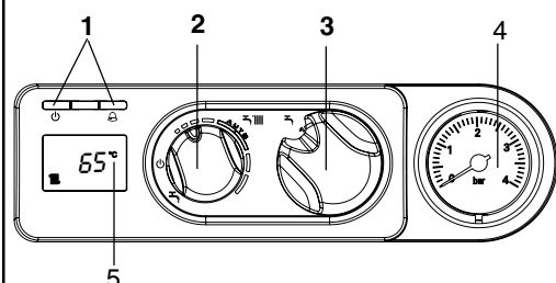
Visualizzatore digitale (5)
