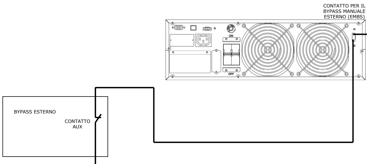
Figura 7 - Collegamento tra BYPASS ESTERNO e contatto EMBS
