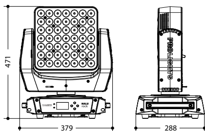
Disegno tecnico
