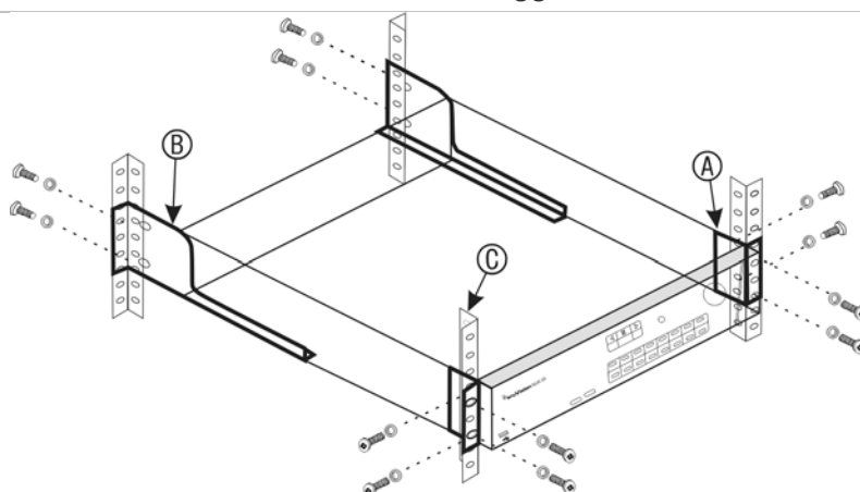
Figura 2: Installazione dell'unità TVN 10 con montaggio a rack
