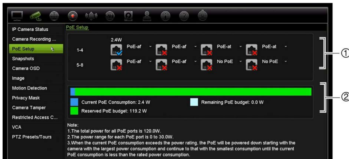
Figura 20: Informazioni su budget energetico PoE per telecamere IP
