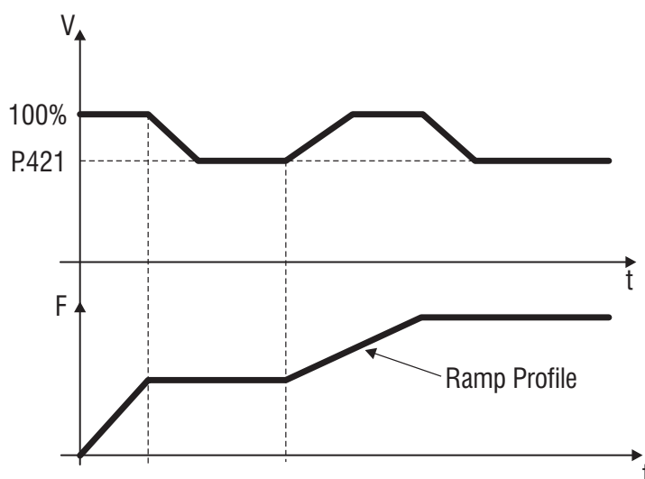
Figura 1.1-33.: Riduzione della tensione d'uscita con P.420 = 1
