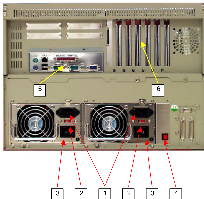
Figura 1.2 - Visione Pannello Posteriore
