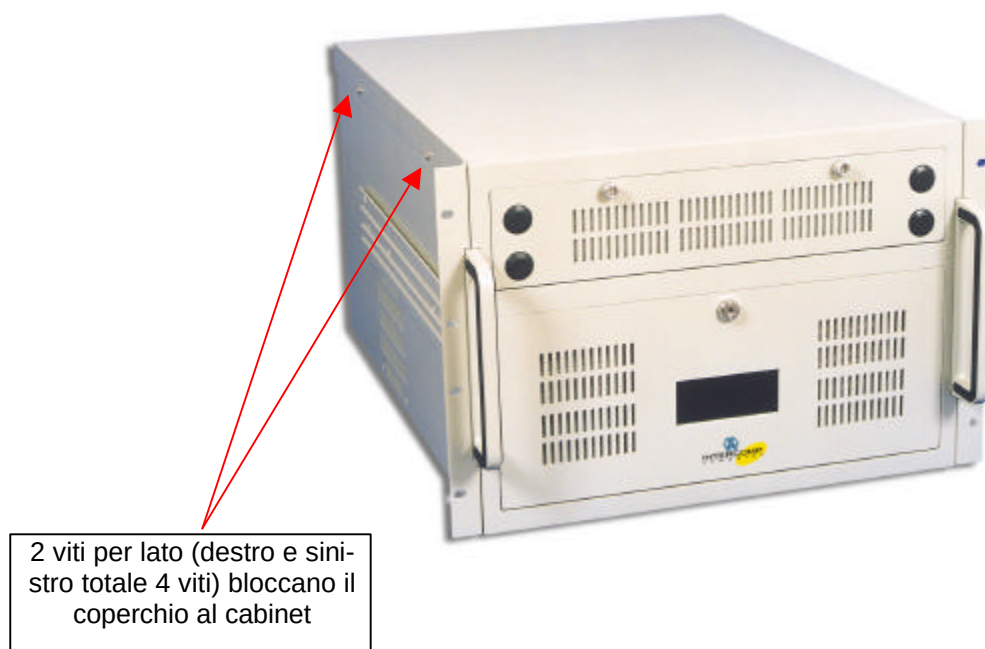
Figura 4. Posizione delle viti per l'apertura o la chiusura del computer (totale 4 viti).
