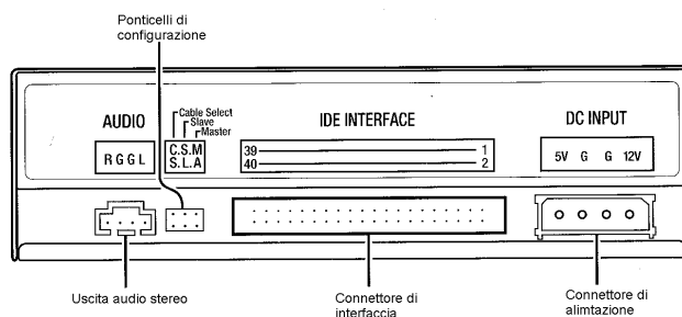
Figura 9. Nella figura sono descritti i connettori posti sul lato posteriore del CD-ROM.
