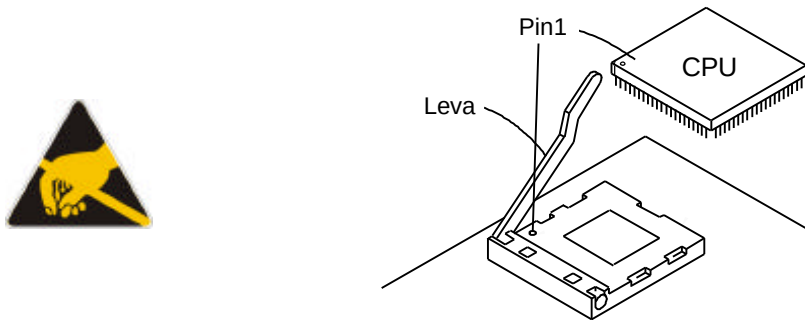
Figura 5. Inserimento della CPU
