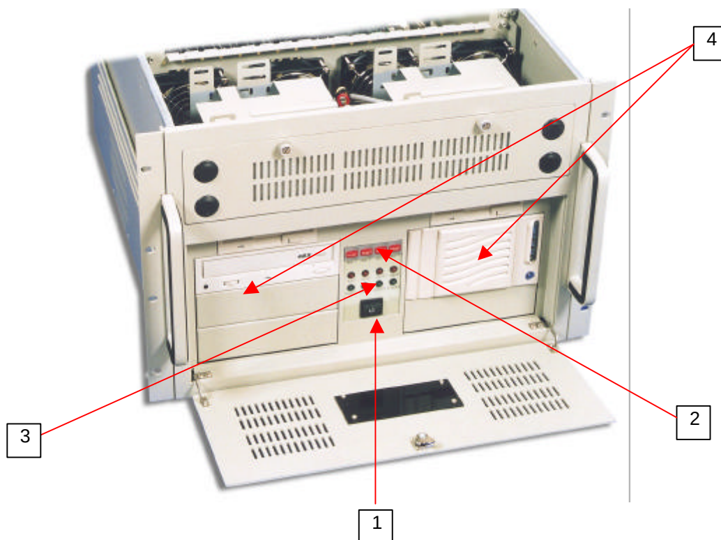
Figura 1.1 - Visione Pannello Frontale
