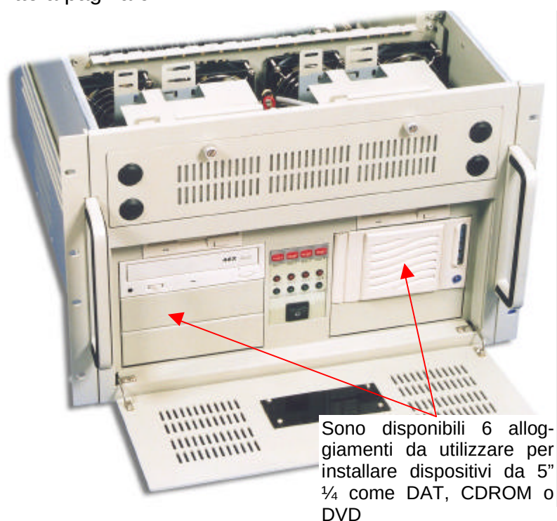
Figura 7. Installazione dispositivo nell'alloggiamento da 5.25"
