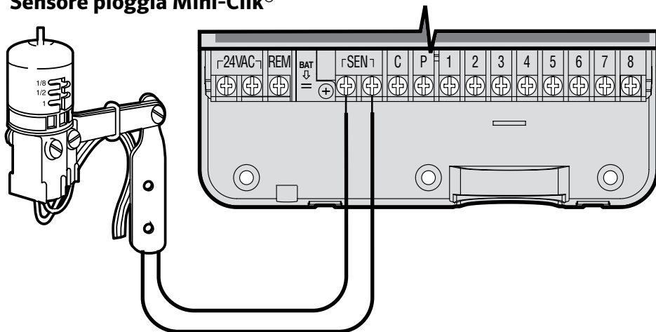
Sensore pioggia Mini-Clik®
