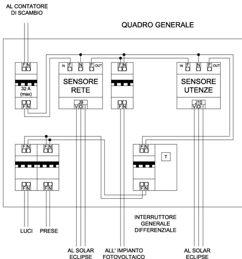
Figura 7 – Schema cablaggio quadro elettrico
