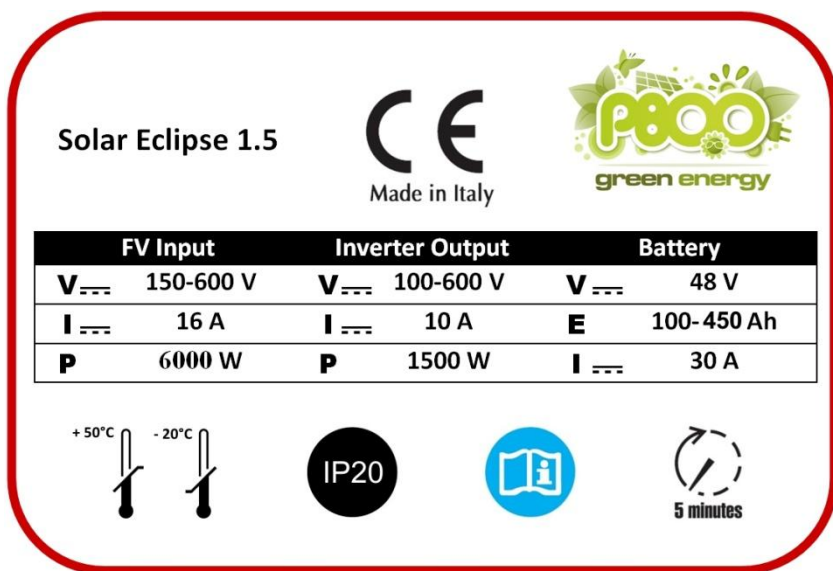
Figura 2 – Targhetta di identificazione e omologazione
