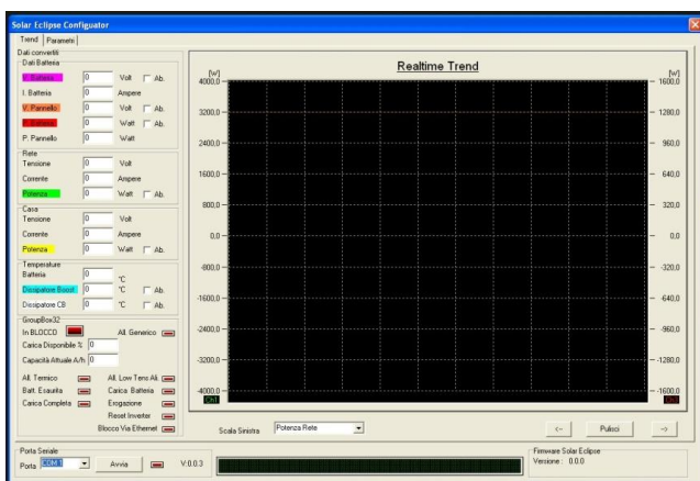
Figura 11 – Software di configurazione – Schermata Trend
