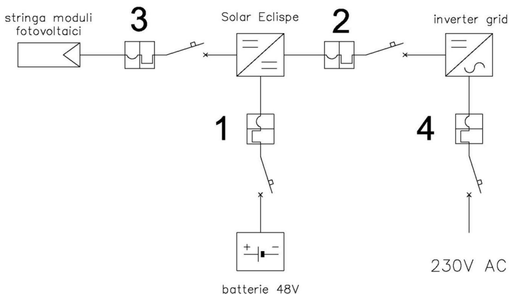
Figura 13 - Schema ordine chiusura/apertura sezionatori avvio/arresto
