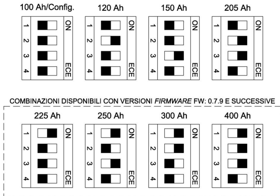
Figura 10 – Configurazione batterie tramite dip-switch
