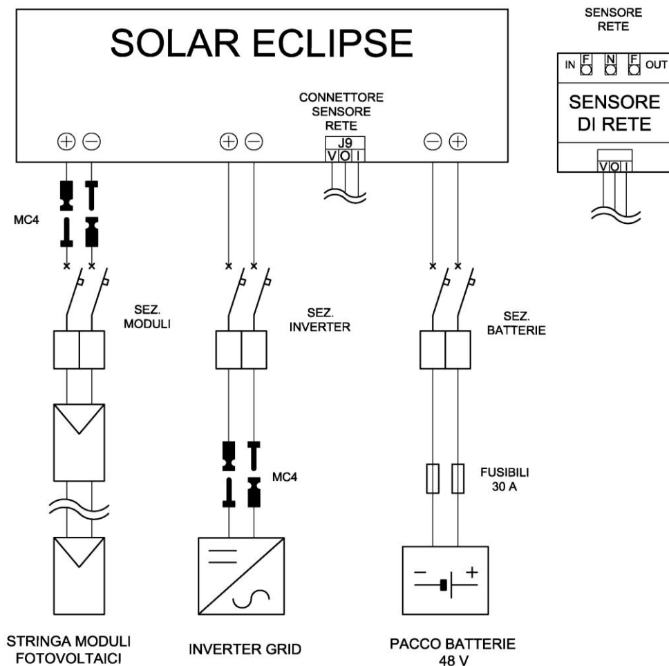
Figura 5 – Schema cablaggio di potenza
