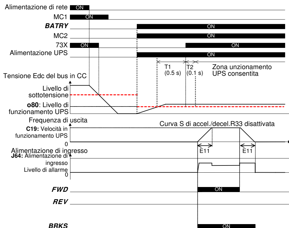
Figura 7.2 Operazione di recupero: diagramma delle temporizzazioni
