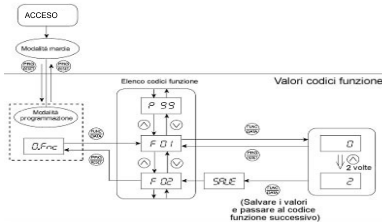
Figura 5.2 Procedura di impostazione funzione
