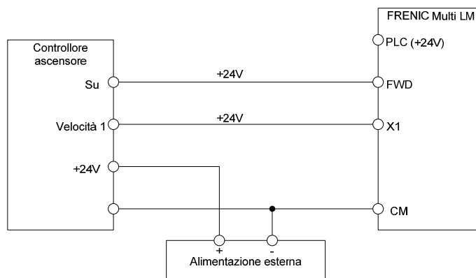
Figura 4.9 Collegamento ad alimentazione esterna
