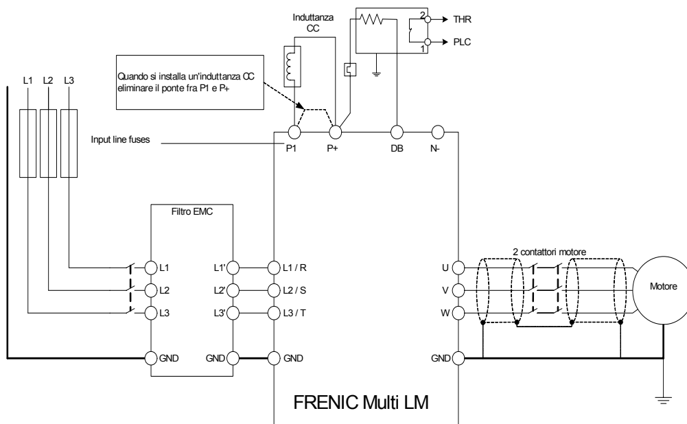
Figura 4.6 Collegamenti dei morsetti del circuito principale
