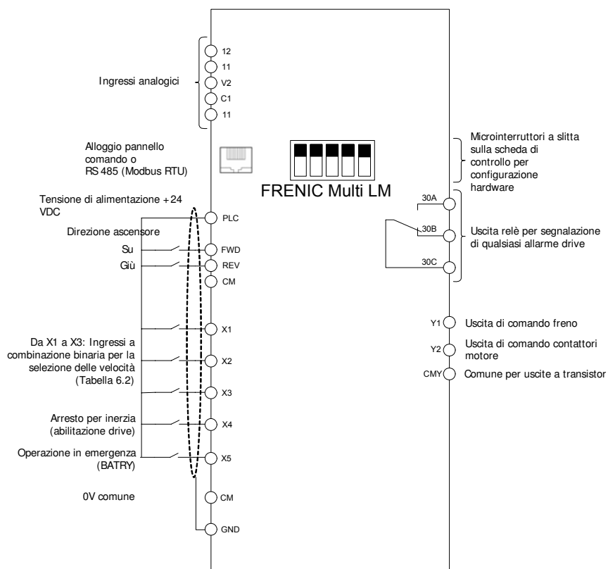
Figura 4.7 Collegamenti dei morsetti di comando
