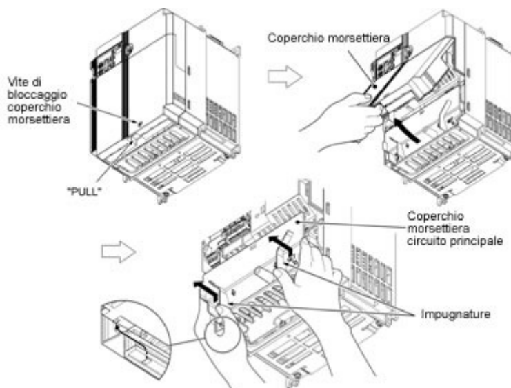
Figura 4.2 Come togliere i coperchi (per inverter con potenza di 5.5 kW e 7.5 kW)
