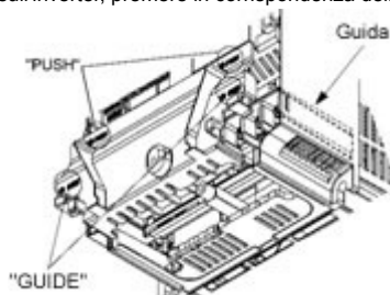
Figura 4.5 Montaggio del coperchio della morsettiere del circuito principale (per inverter con potenza di 11 kW e 15 kW)
