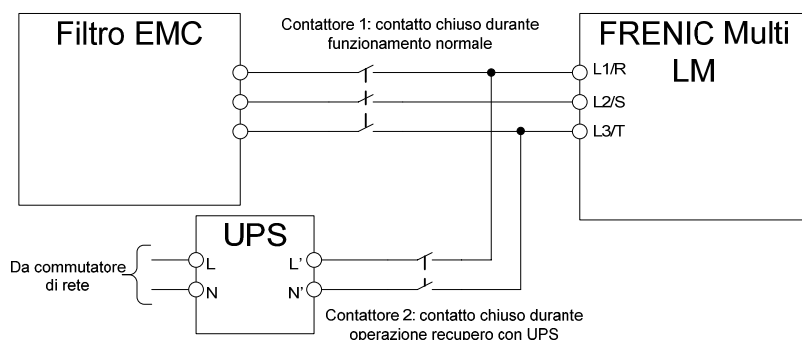
Figura 7.1 Schema cablaggio di base
