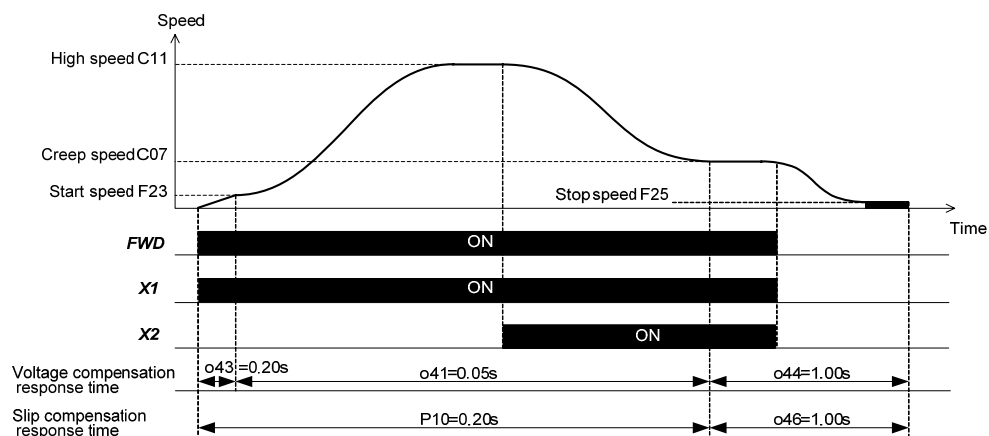
Figura 7.3 funzionamento in Normale
