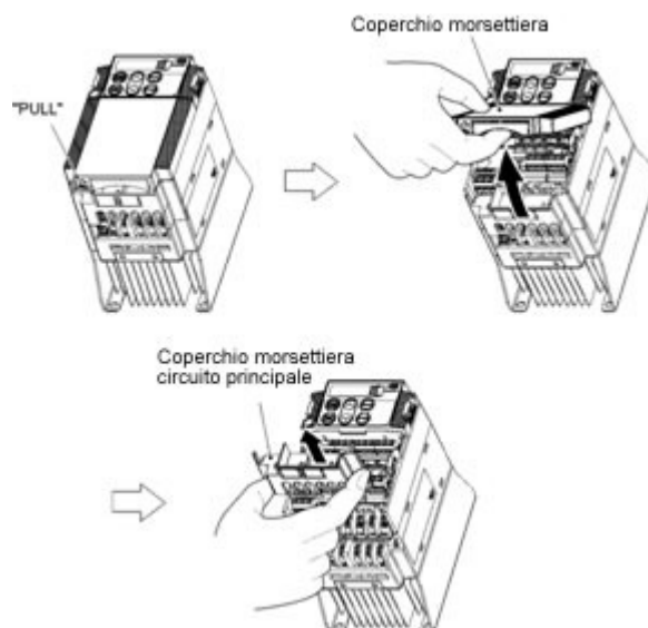
Figura 4.1 Come togliere i coperchi (per inverter con potenza inferiore a 5.5 kW)
