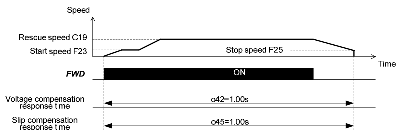
Figura 7.4 Funzionamento in Emergenza
