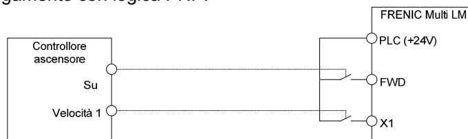
Figura 4.8 Collegamento normale utilizzando i contatti disponibili del controller ascensore
