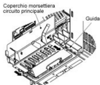
Figura 4.3 Montaggio del coperchio della morsettiere del circuito principale (per inverter con potenza di 5.5 kW e 7.5 kW)
