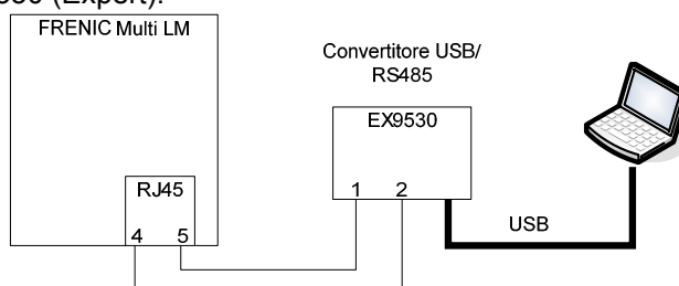
Figura 4.12: Collegamento di FRENIC Loader2 con un PC
