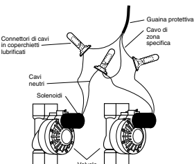
FIGURA 17: Collegamento dei cavi del timer alle valvole
