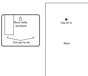
FIGURA 15: Installazione di un timer per interni
