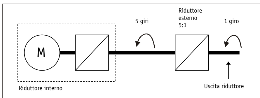
Fig. 7: riduttore esterno
