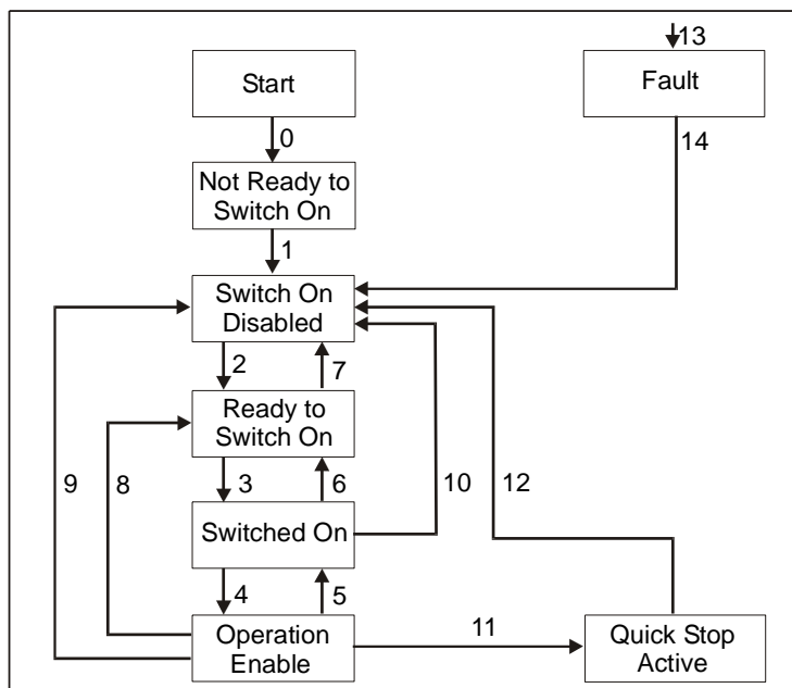
Fig. 10: macchina a stati
