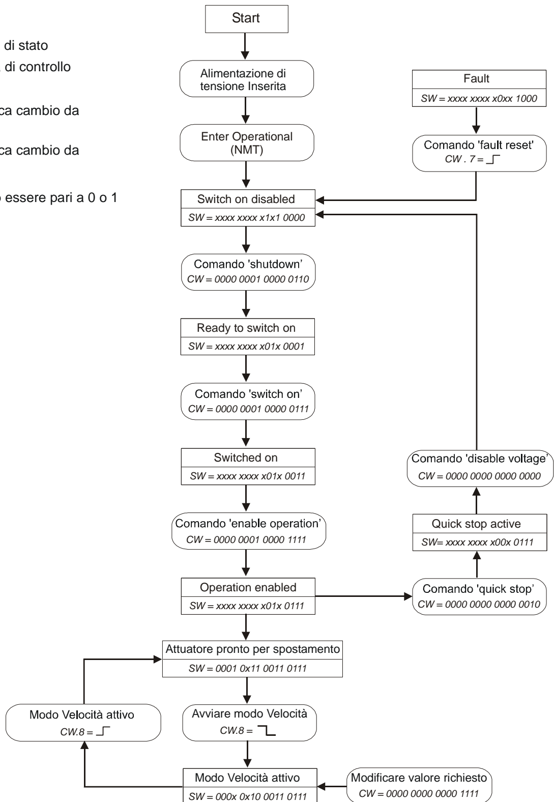
Fig. 12: flow chart modo operativo Profile Velocity Mode (modo Velocità)
