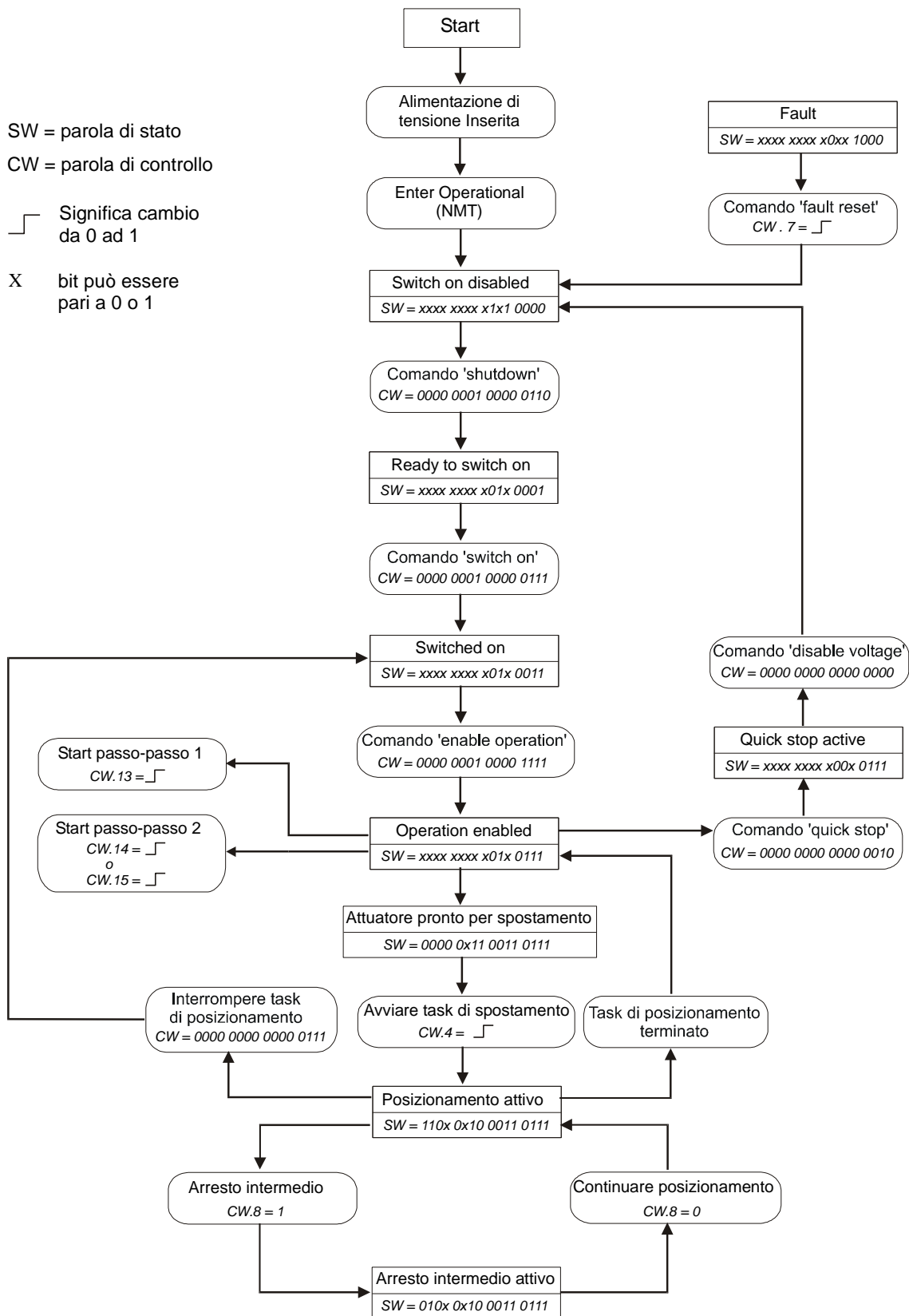
Fig. 11: flow chart modo operativo Profile Position Mode (modo Posizionamento)
