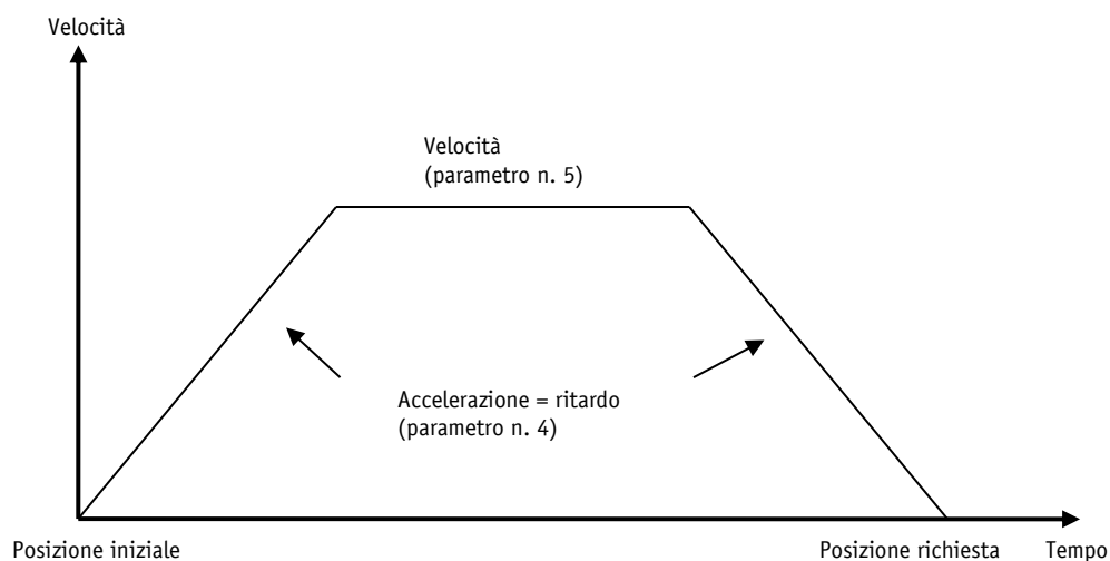
Fig. 3: rampa con modo Posizionamento diretta
